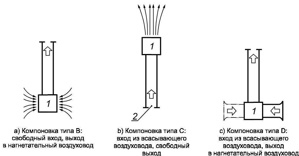
Рисунок С.1 — Компоновки вентилятора с воздуховодами
