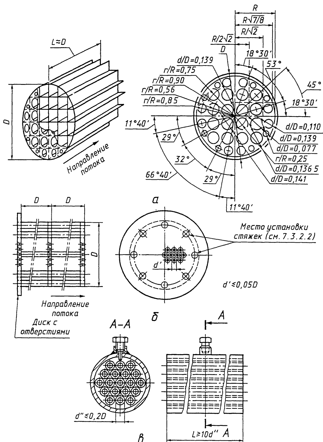
Рисунок 1 – Струевыпрямители
