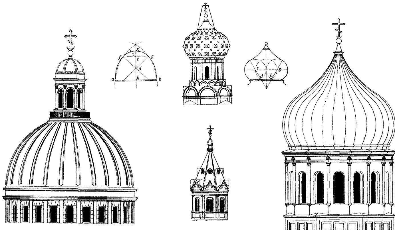
Рис. 55. Разновидности глав храмов (из альбома А. Красовского, 1854 г.)
