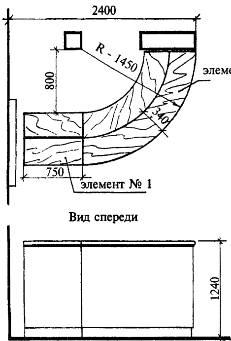
Общий вид прилавка сверху
