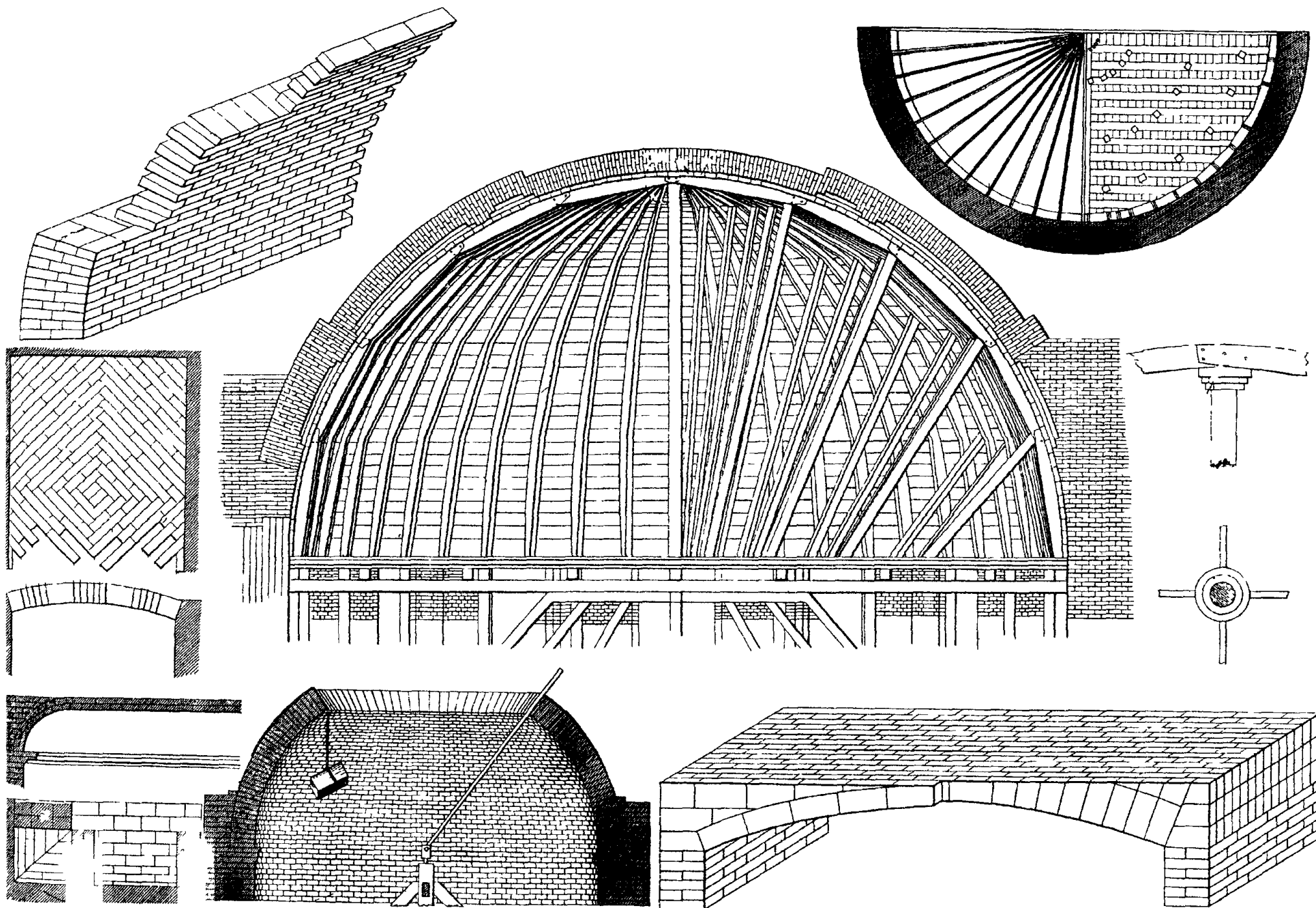
Рис. 50. Своды (из альбома А. Красовского, 1904-1911)
