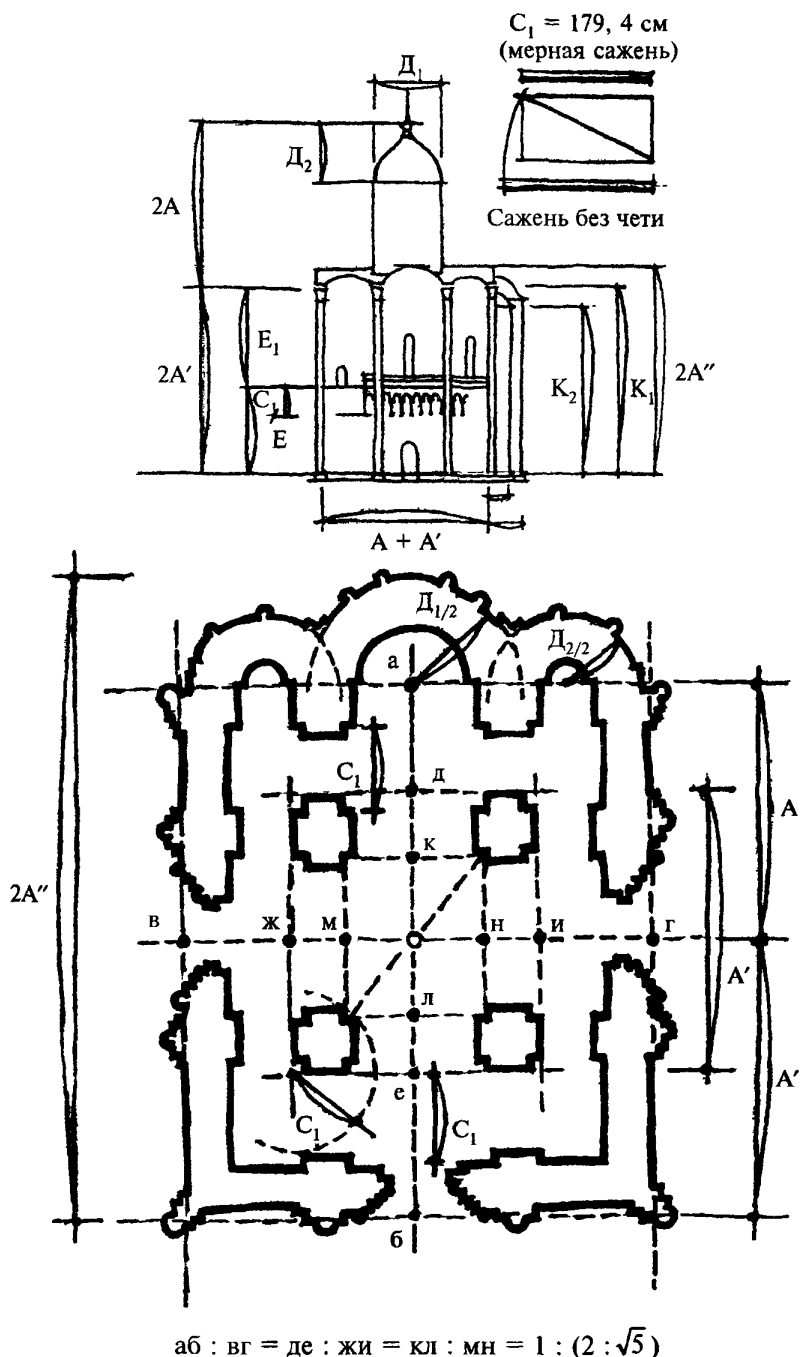
Рис. 16. Соразмерности храма Покрова на Нерли
