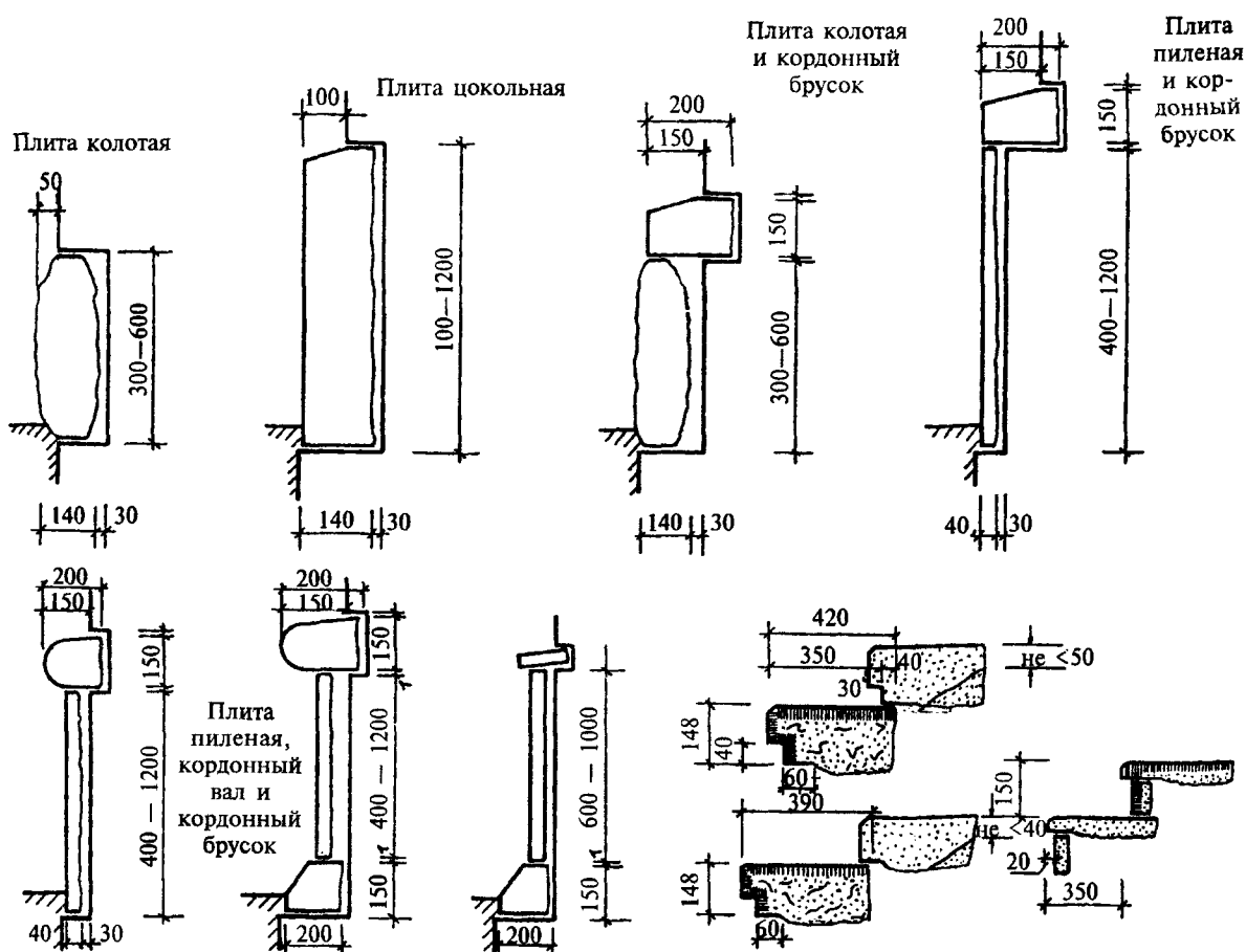
Рис. 31. Примеры применения облицовки в цоколе и на лестницах
