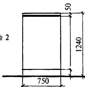
Вид со стороны продавца (откидная дверка не показана)
