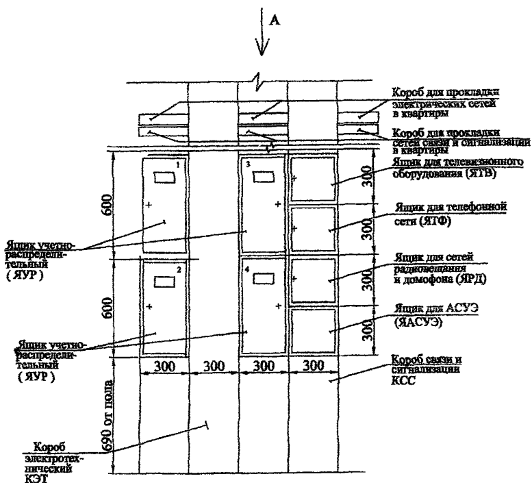
Вид А
