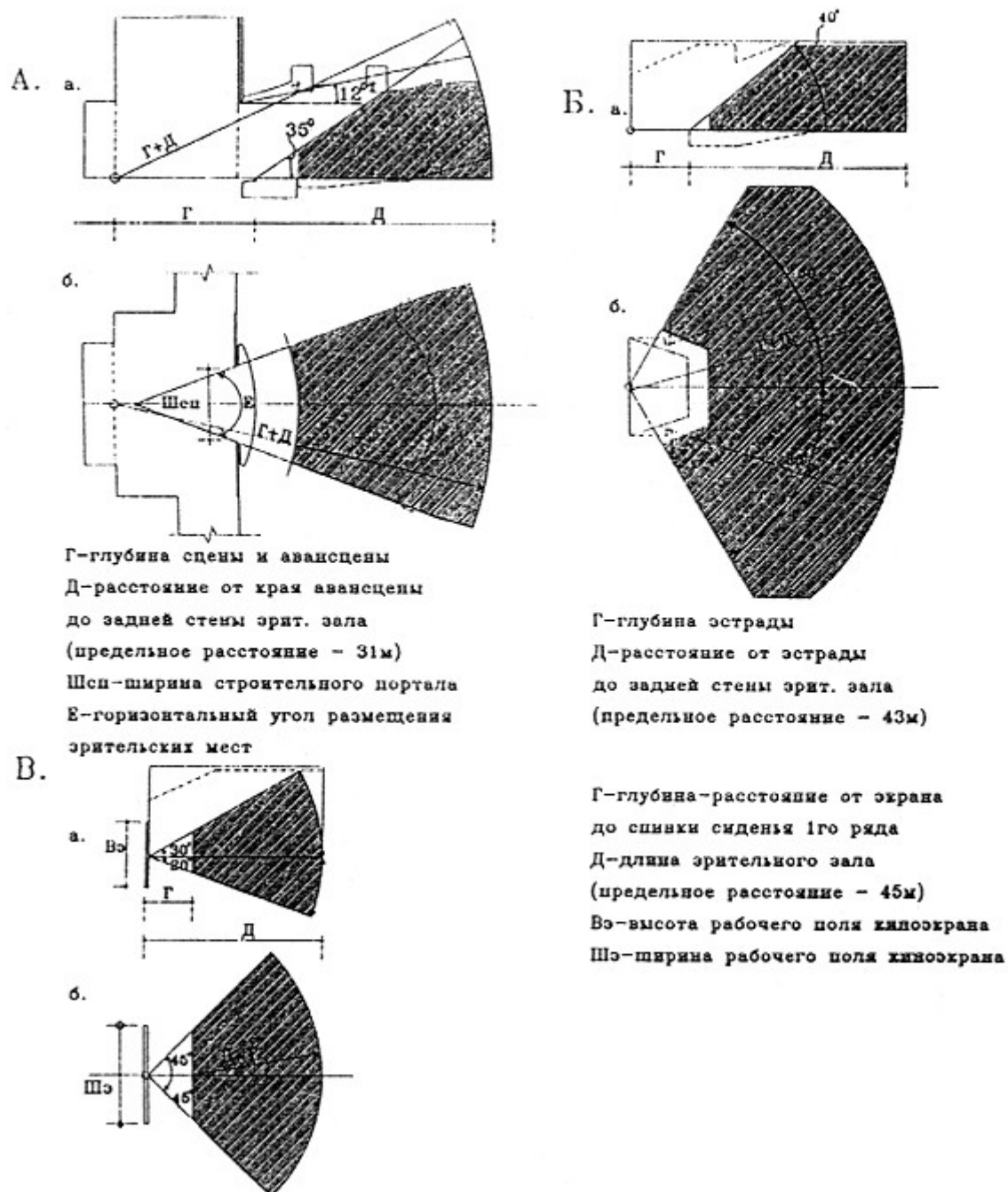
Рис.3. Зоны оптимальной видимости - зоны расположения зрителей А - перед сценой, Б - перед эстрадой; В - перед киноэкраном; а - разрез, б - план
