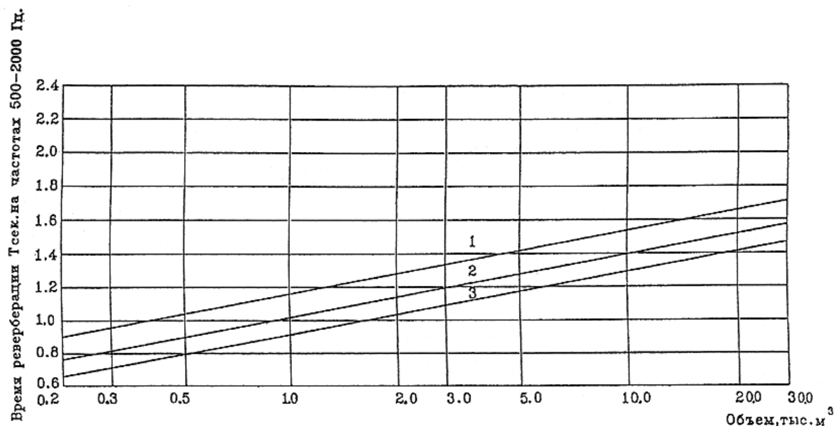
Рисунок 4. Рекомендуемое время реверберации на частотах 500-2000 Гц для залов различного назначения в зависимости от их объема
