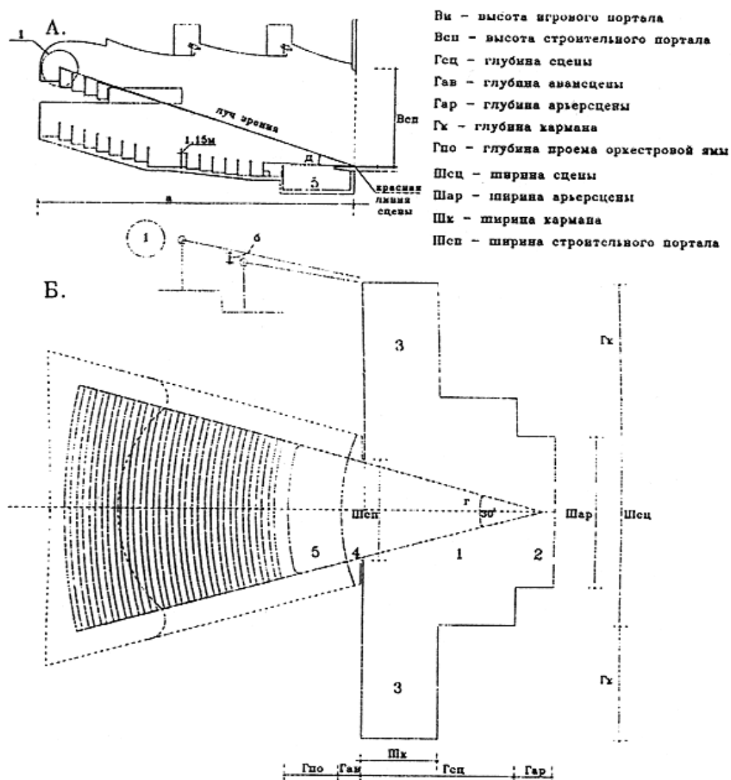
Рис.2. Расчетные параметры зрительных залов с колосниковой глубинной портальной сценой
