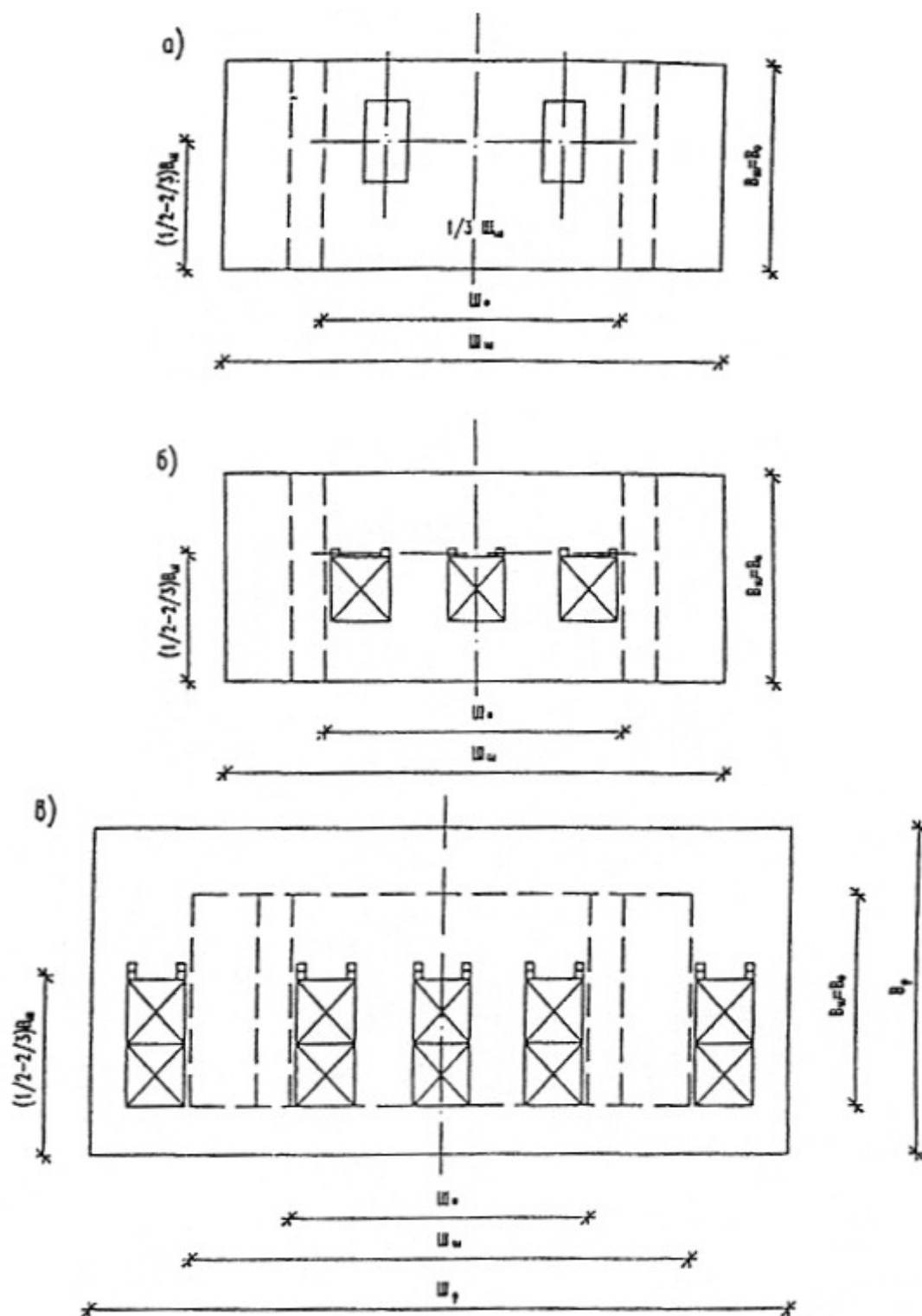
Схемы размещения двух (а), трех (б), пяти (в) заэкранированных громкоговорителей.
