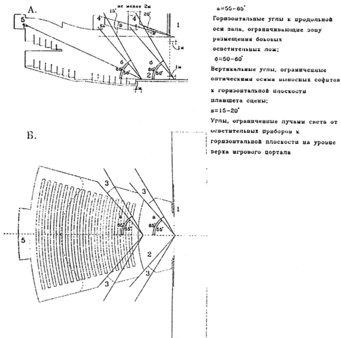
Рис.5. Схема размещения помещений постановочного освещения сцены
