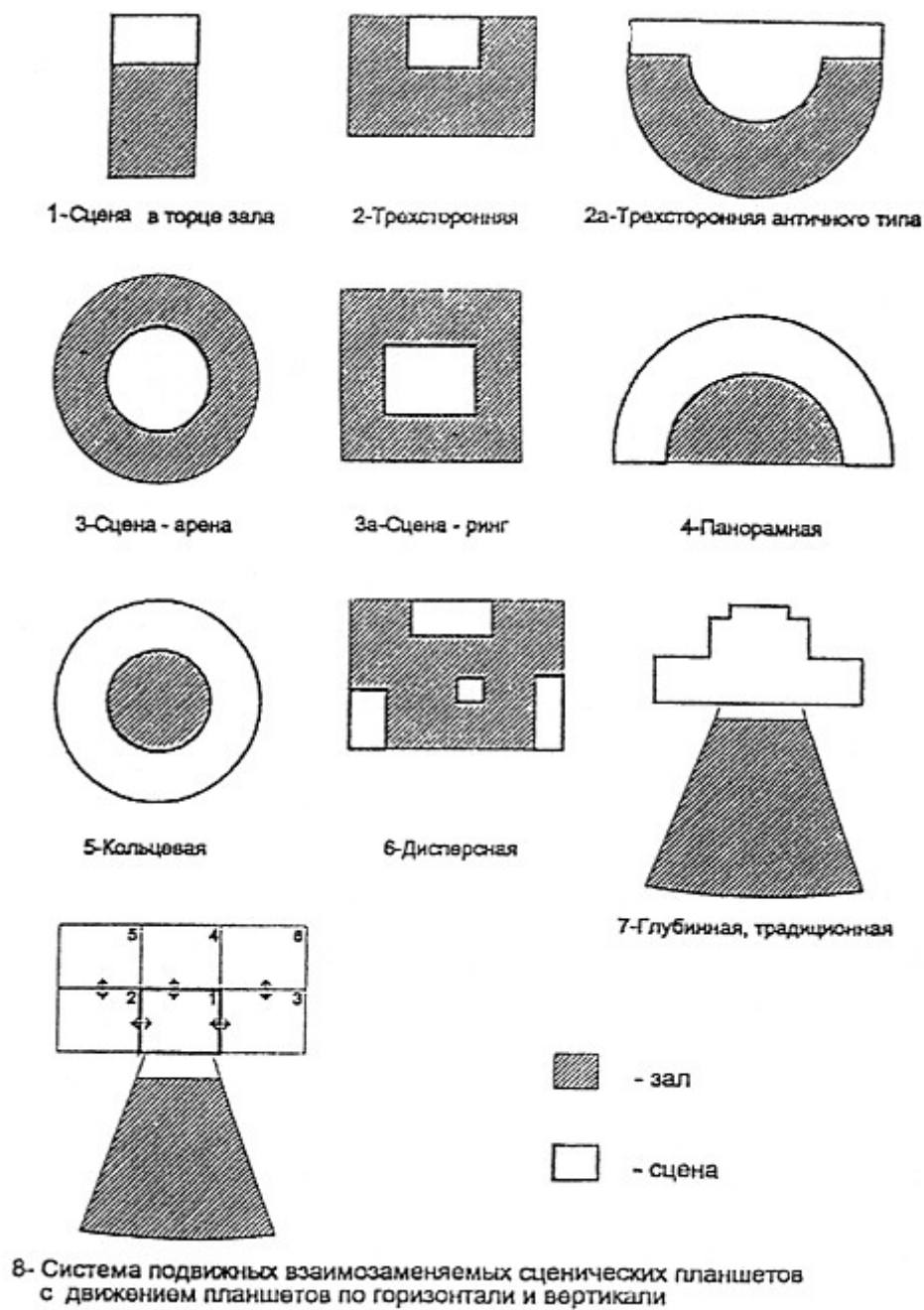
Рис.1. Типы сцен. Схемы взаимосвязи зала и сцены
