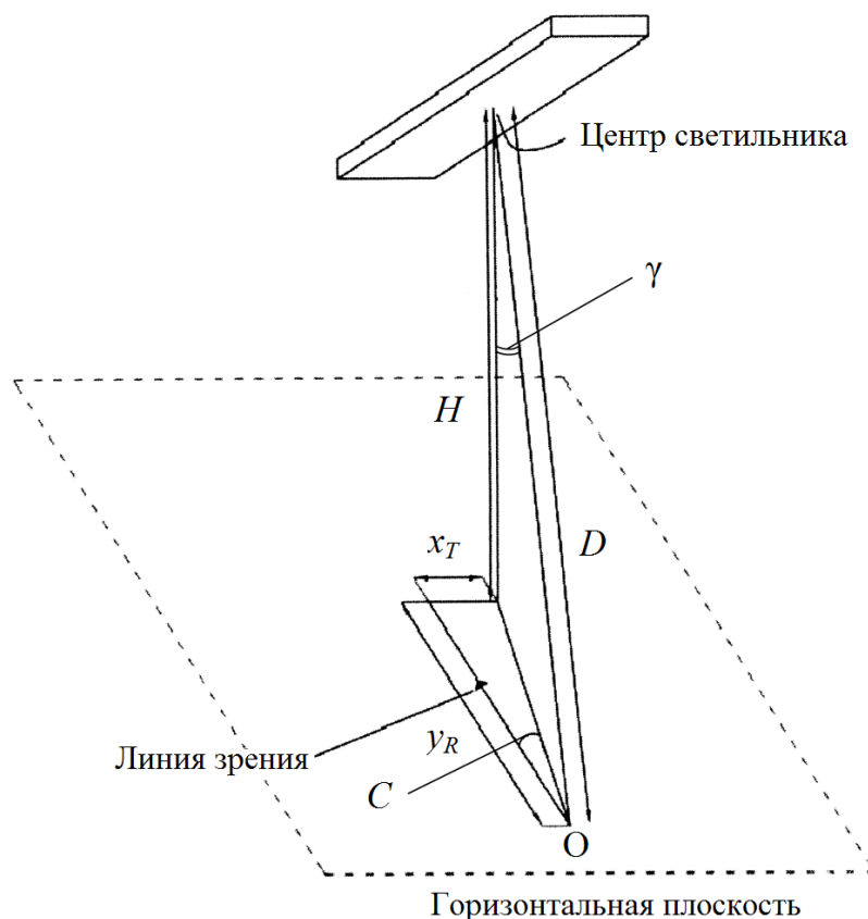
Рисунок 2.1 – Расположение центра светильника относительно работающего
