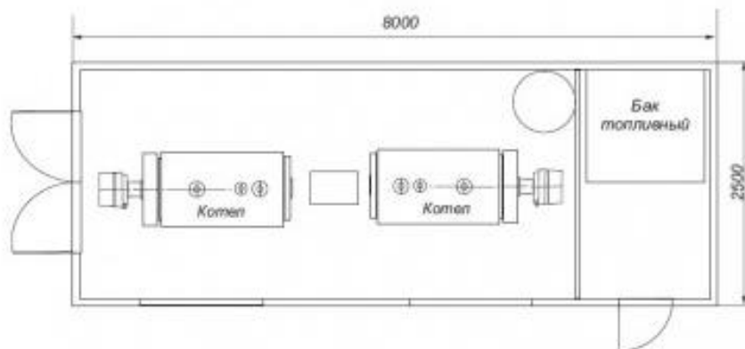
Рисунок 5.2 – Котельная
