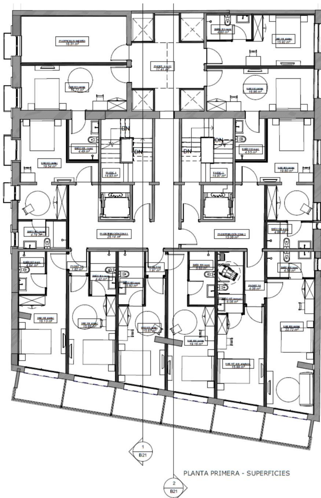
Рисунок Д.1 – Второй этаж гостиничного комплекса
