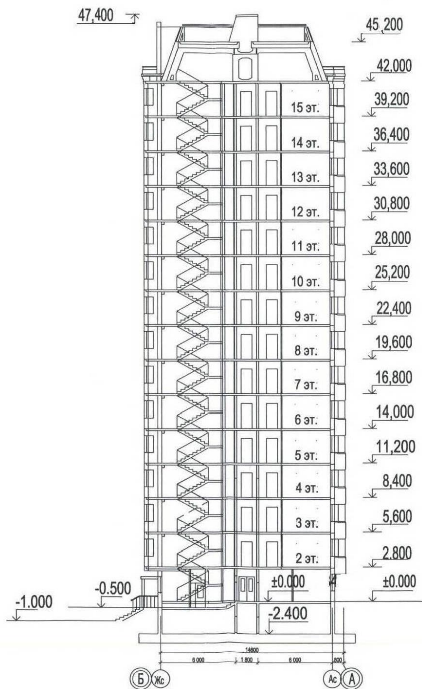
Рисунок Б.4 – Разрез типового жилого дома П44
