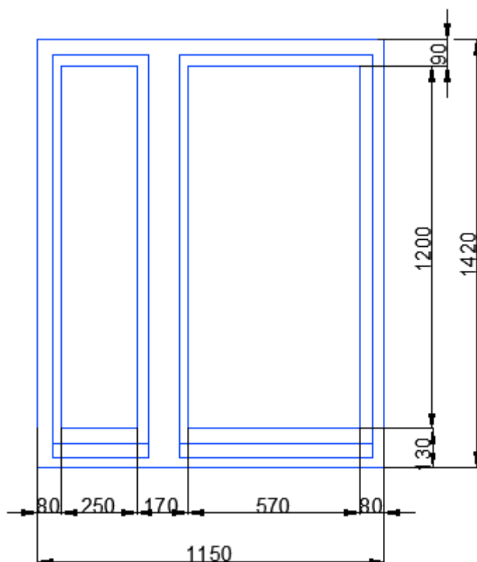
Рисунок 5.6 – Оконный блок с двухкамерным стеклопакетом, обозначенный О-4
