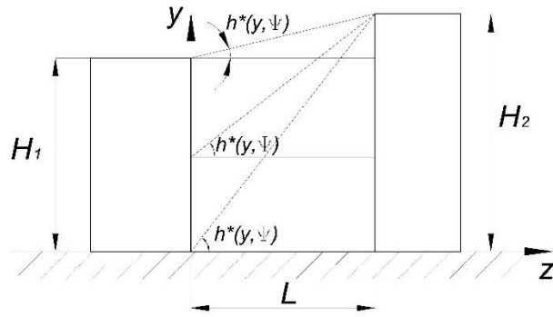
Рисунок 5.2 – Схема расположения зданий в разрезе.
