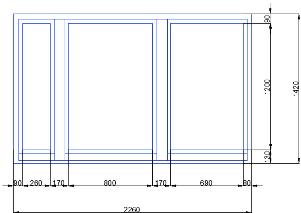
Рисунок 5.4 – Оконный блок с двухкамерным стеклопакетом, обозначенный О-1
