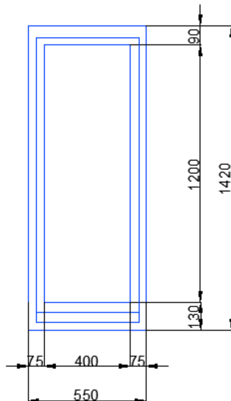
Рисунок 5.6 – Оконный блок с двухкамерным стеклопакетом, обозначенный О-4
