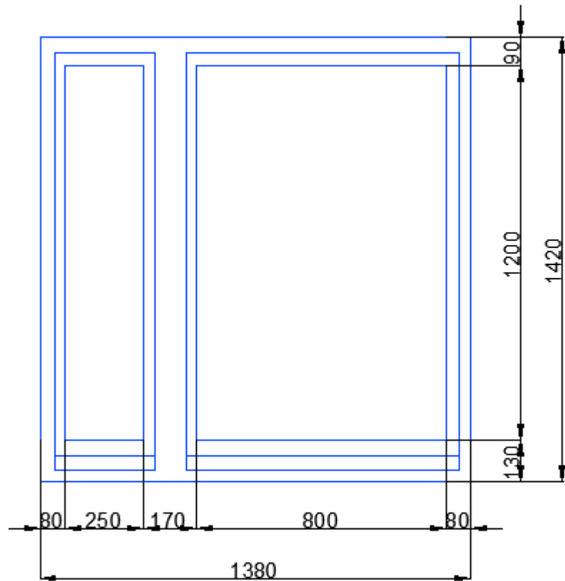
Рисунок 5.4 – Оконный блок с двухкамерным стеклопакетом, обозначенный О-1
