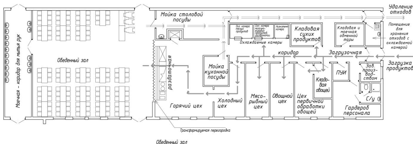
Рисунок 9.2 – Схема взаимного размещения помещений столовой
