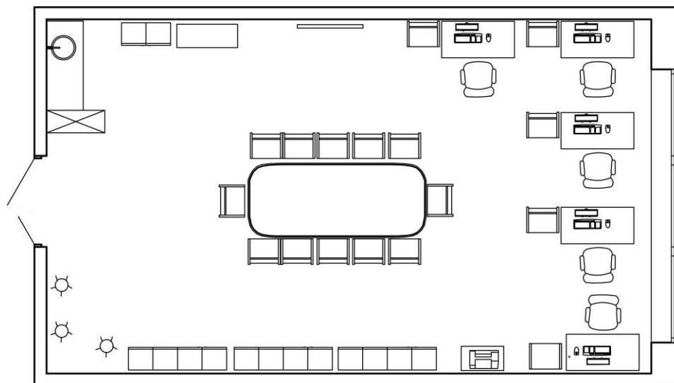
Рисунок 9.3 – Расстановка оборудования в учительской - методическом кабинете
