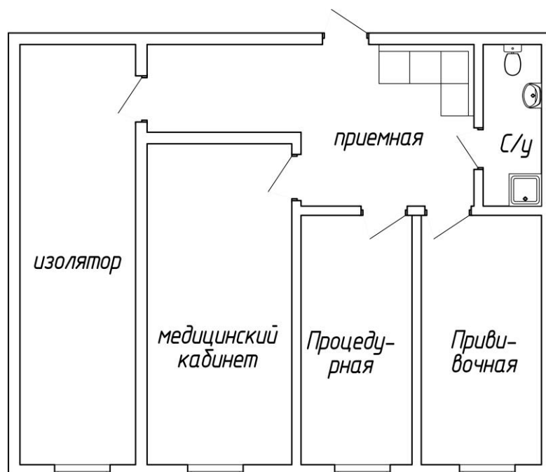
Рисунок 9.3 – План-схема помещений медицинского блока
