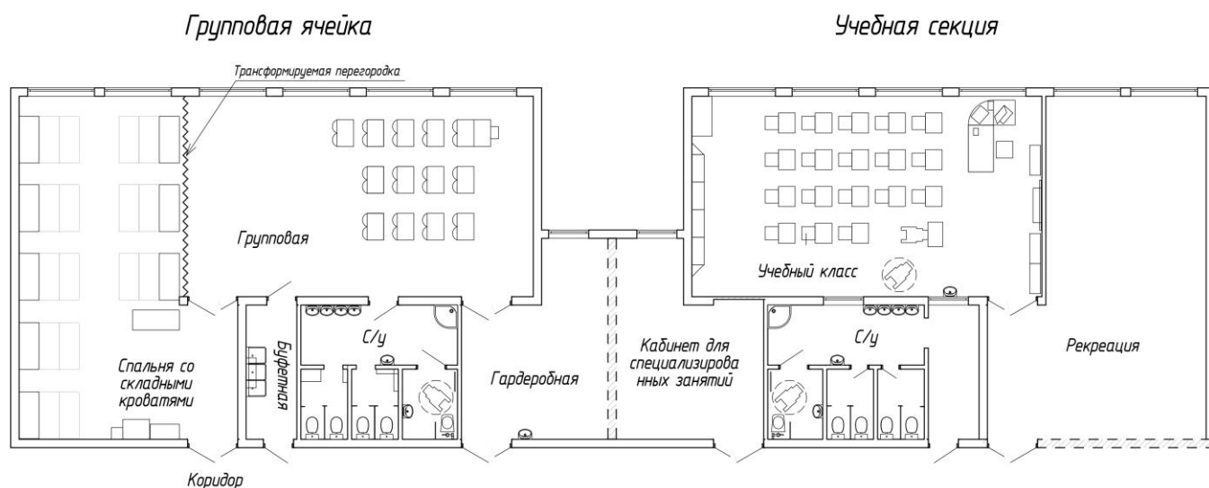
Рисунок 8.2 – Трансформация групповой ячейки и гардеробной
