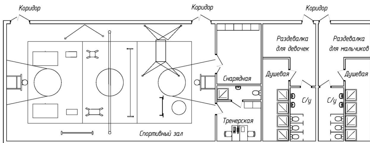
Рисунок 9.1 – Схема помещений спортивного зала КБНК
