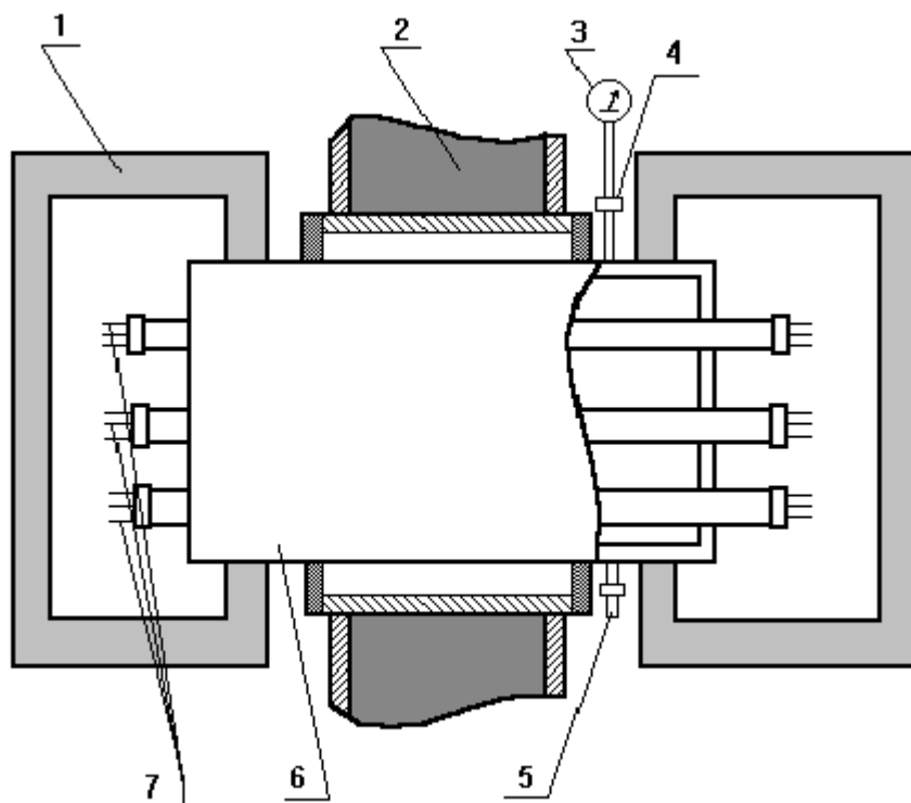
Рис. 2. Схема герметичного кабельного ввода:
