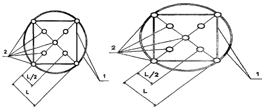
Схема расположения модельных очагов пожара:
