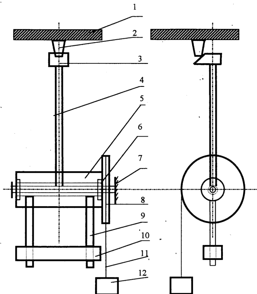
Схема устройства для проверки устойчивости радиоизотопных извещателей к прямому механическому удару (удар молотком):
