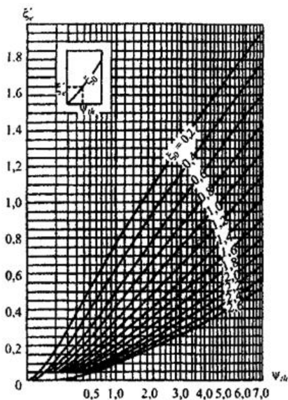
Рисунок К.6 - Графики для определения коэффициента \xi'_e
