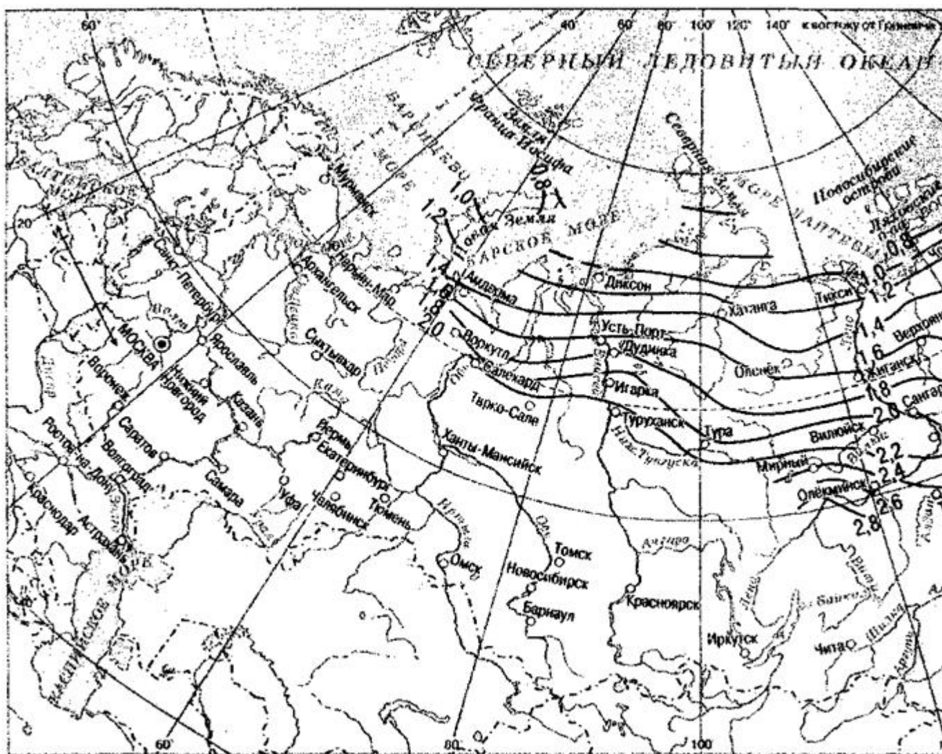
Рисунок Г.2 - Глубины оттаивания глинистых грунтов
