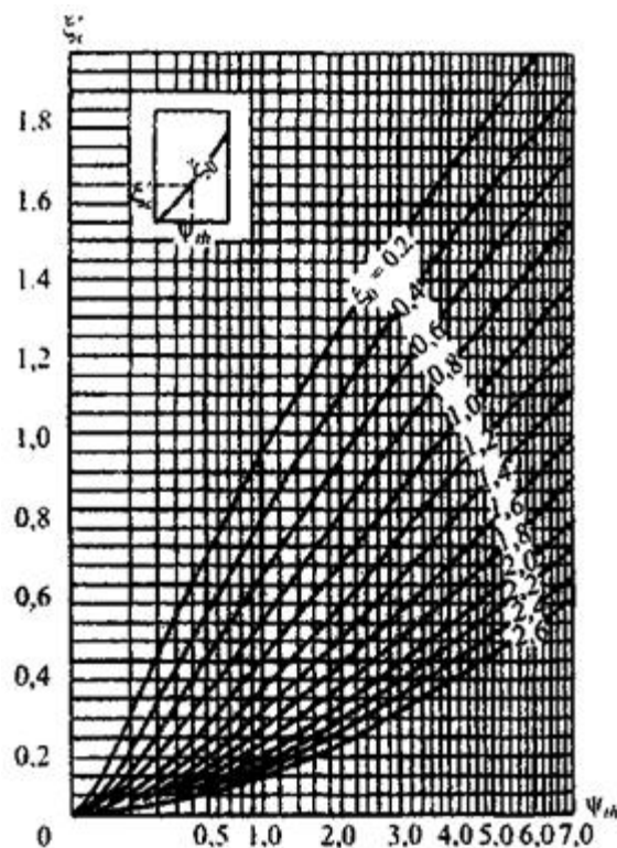
Рисунок К.5 - Графики для определения коэффициента \xi'_c
