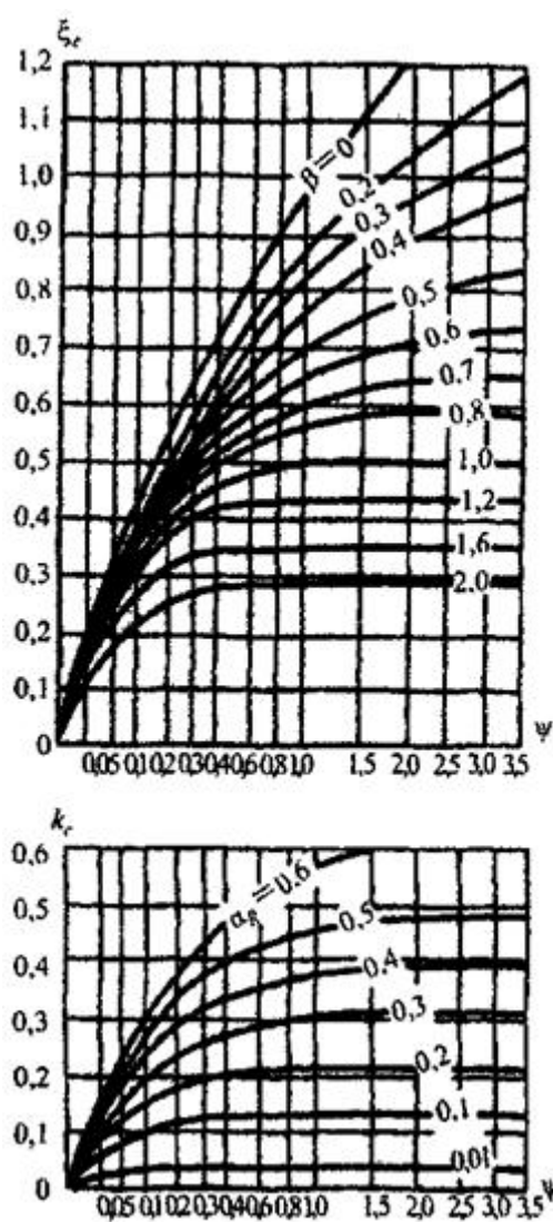
Рисунок К.1 - Графики для определения коэффициентов \xi_c и k_c
