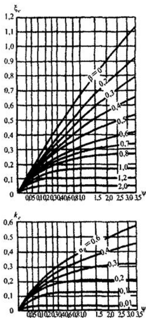
Рисунок К.2 - Графики для определения коэффициентов \xi_e и k_e
