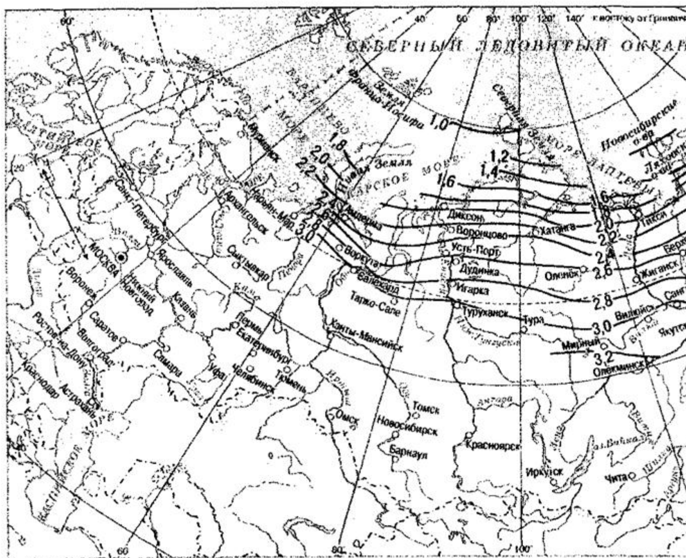
Рисунок Г.1 - Глубины оттаивания песчаных грунтов
