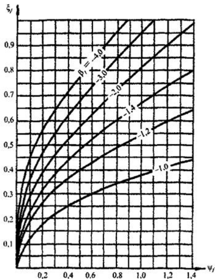
Рисунок Е.1 - Графики для определения коэффициента \beta_f
