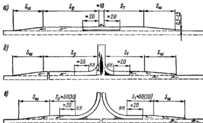
a – В зоне автобусных остановок; б – На пересечениях; в – На самостоятельных съездах и въездах
