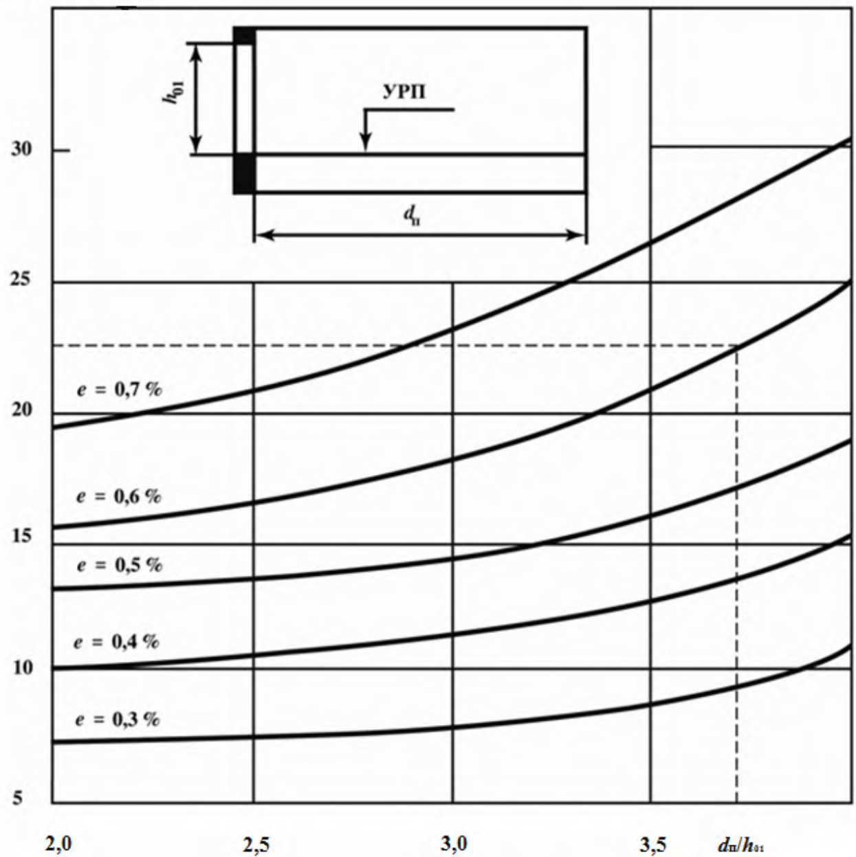
Рисунок 8.1 – График для определения относительной площади световых проемов S_{c.o}/S_{\Pi} при боковом освещении в жилых помещениях
