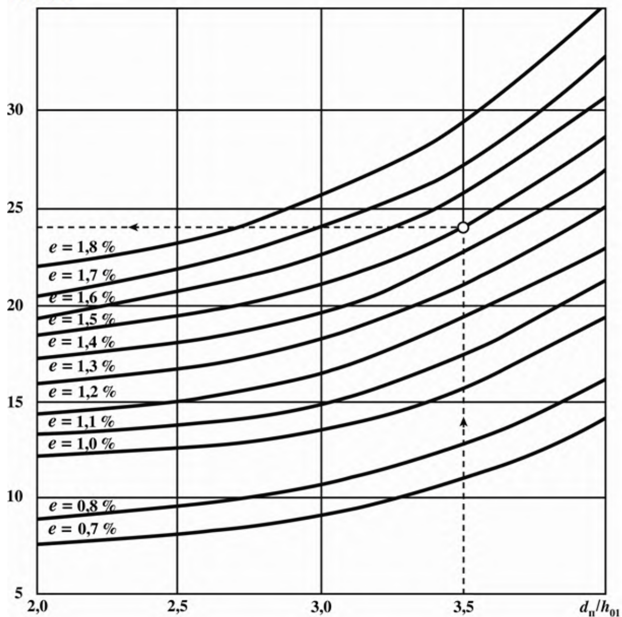
Рисунок 8.3 – График для определения относительной площади световых проемов S_{c.o}/S_n при боковом освещении учебных кабинетов общеобразовательных организаций
