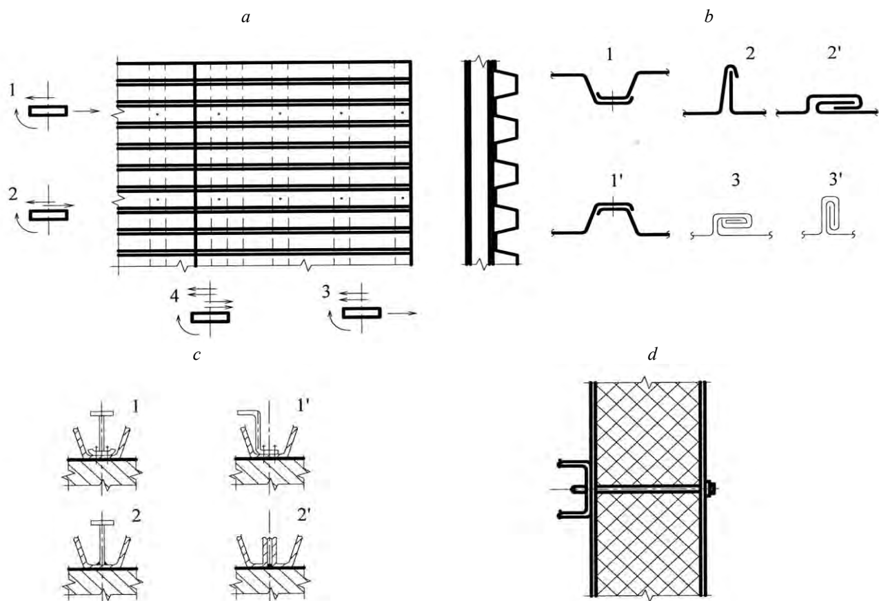
a – фрагмент конструкции покрытия со стальным профилированным настилом и схема действия сил на опорах (1- соединения в среднем участке; 2 и 3- соединения соответственно по продольным и поперечным полкам; 4 – соединения в месте пересечения продольных и поперечных полок); b – схема соединений по продольным полкам (1 и 1' – при расположении полок внахлест в нижнем и верхнем положениях соответственно для утепленных и холодных покрытий; 2 и 2' – простой стоячий и лежащий фальцы; 3 и 3' – двойной фальц, стоячий и лежащий); c – сдвигоустойчивые элементы (1 и 1' – на высокопрочных дюбелях; 2-на контактной сварке; 2' - на дуговой сварке); d – фрагмент трехслойной стеновой панели на самосверлящем винте
