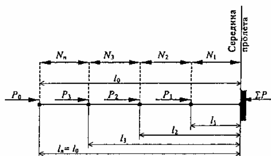
Рисунок Л.1 – Расчетная схема сжатых участков пояса фермы
