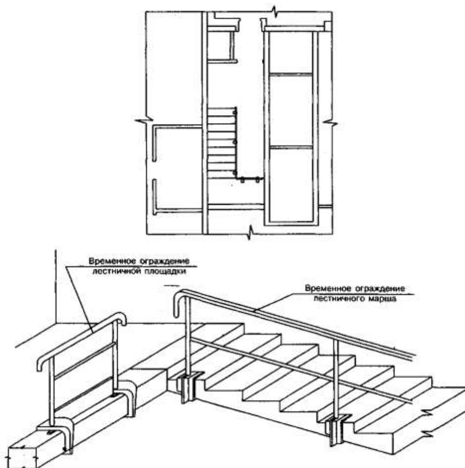
Установка временного ограждения лестничных площадок и лестничных маршей
