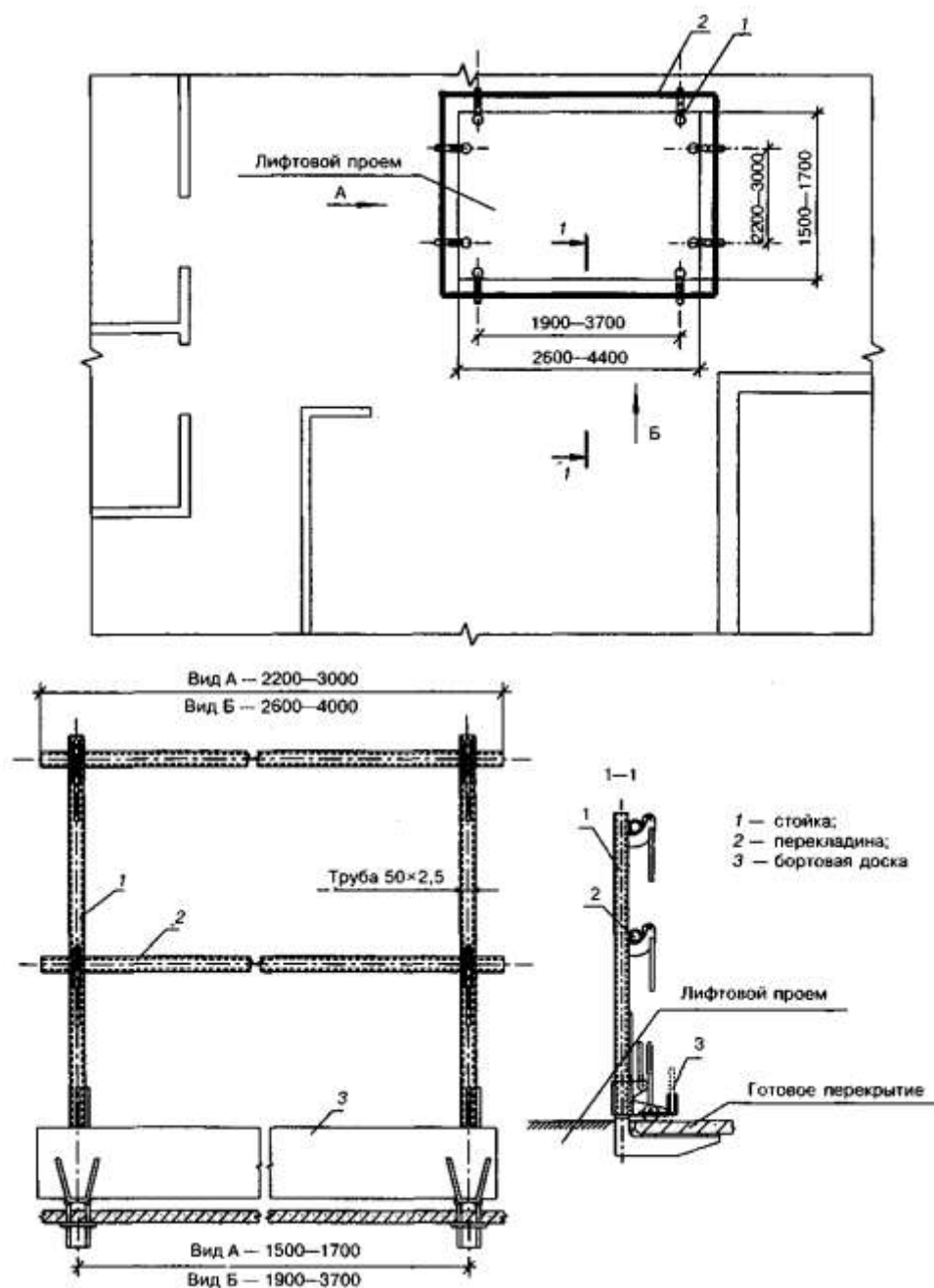
Рисунок 5 — Схема установки временного ограждения лестничной клетки
