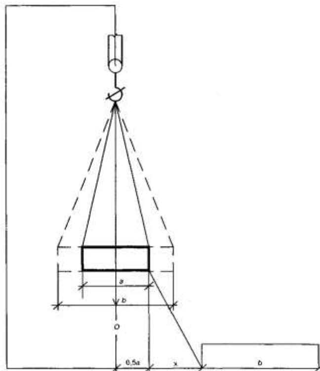
O — граница зоны обслуживания краном; a — наименьший габарит перемещаемого груза;
