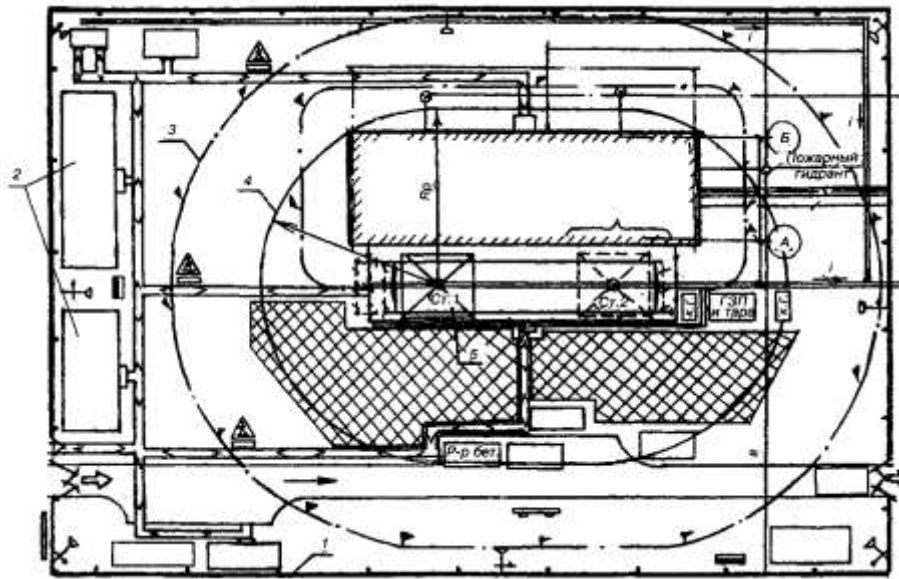
1 — ограждение строительной площадки; 2 — санитарно-бытовые помещения; 3 — граница зоны, опасной для нахождения людей во время перемещения грузов; 4 — граница зоны обслуживания краном; 5 — башенный кран
