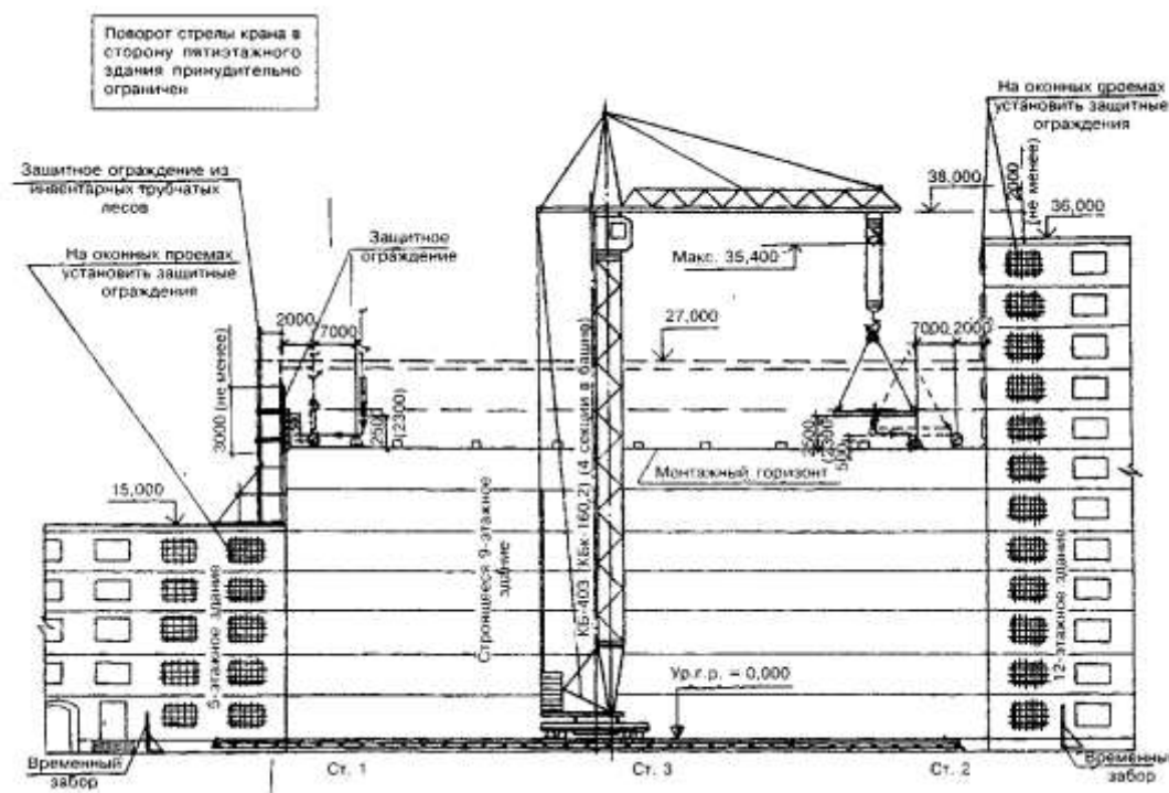
Рисунок 4 — Разрез I—I
