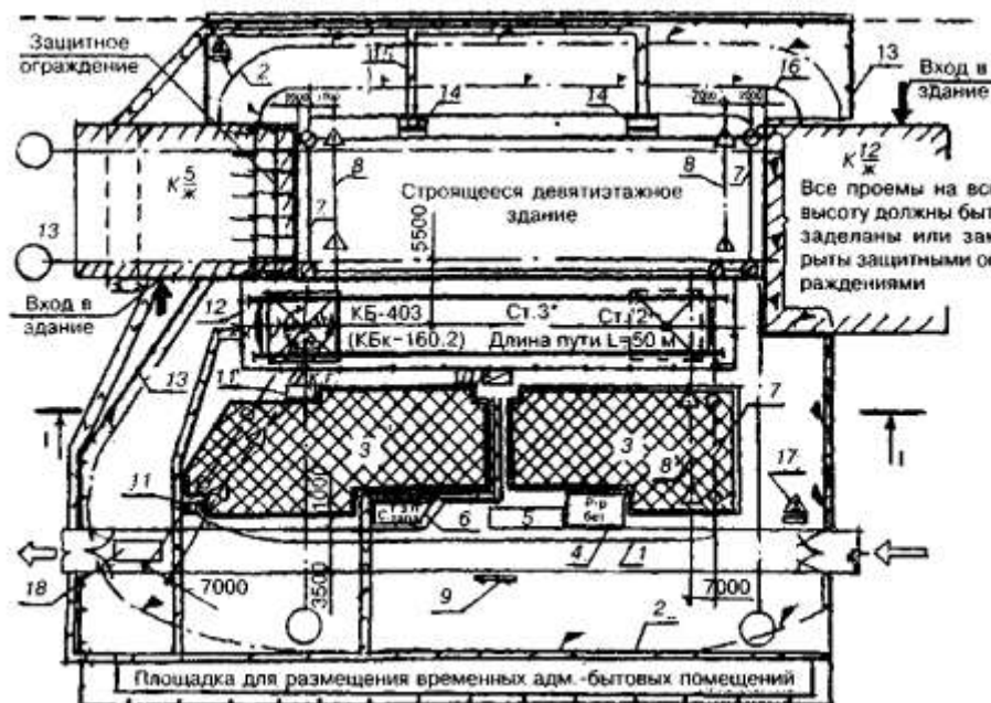
Рисунок 2 — Определение границы опасной зоны перемещаемого краном груза
