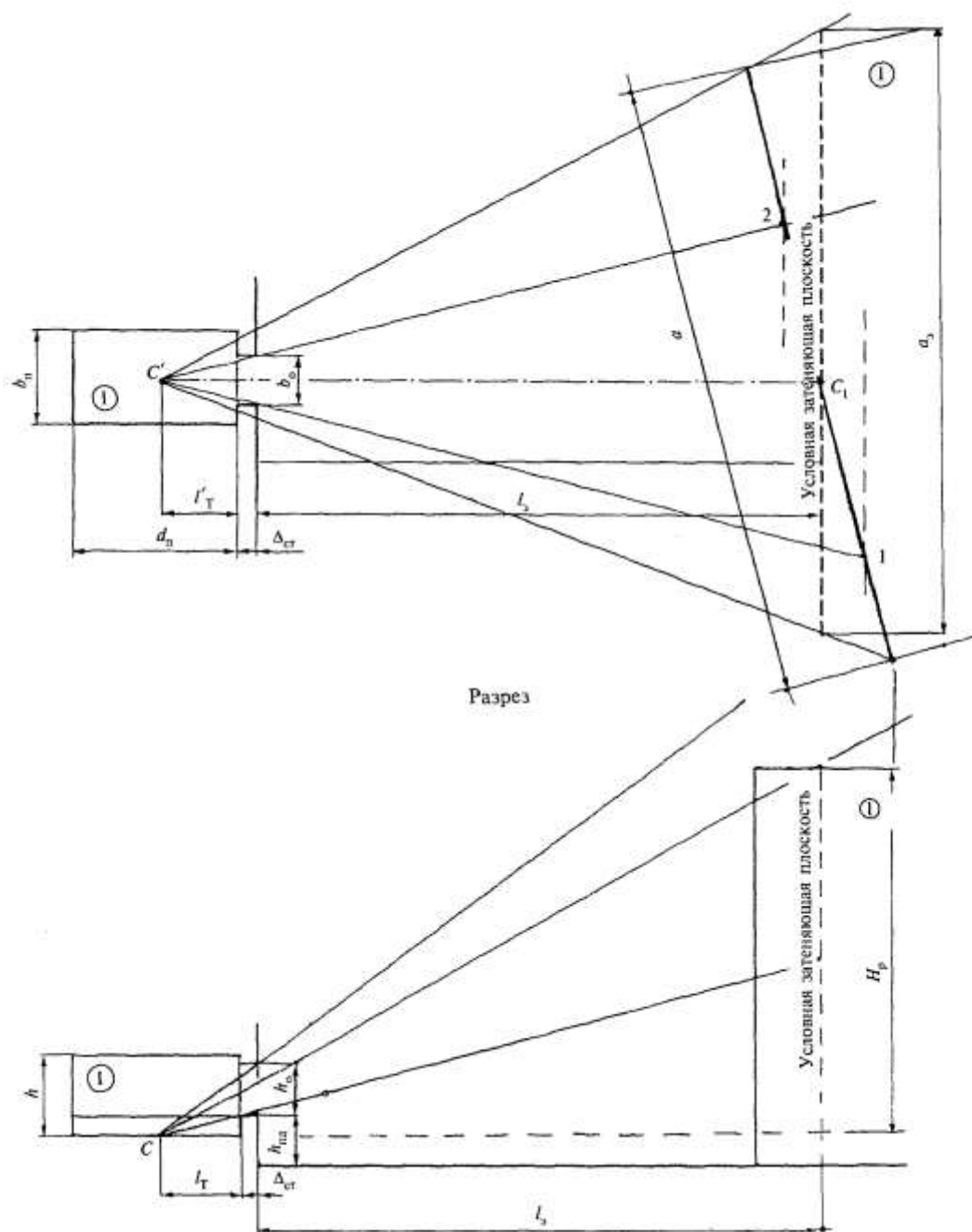
Рисунок Б.2 — Схема № 2 к определению параметров застройки при расположении экранирующего здания под углом к исследуемому зданию
