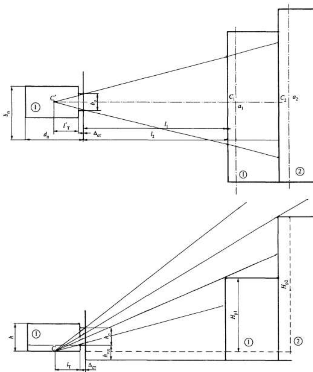
Рисунок Б.7 — Схема № 5 к определению параметров застройки со сложной конфигурацией по высоте экранирующего здания
