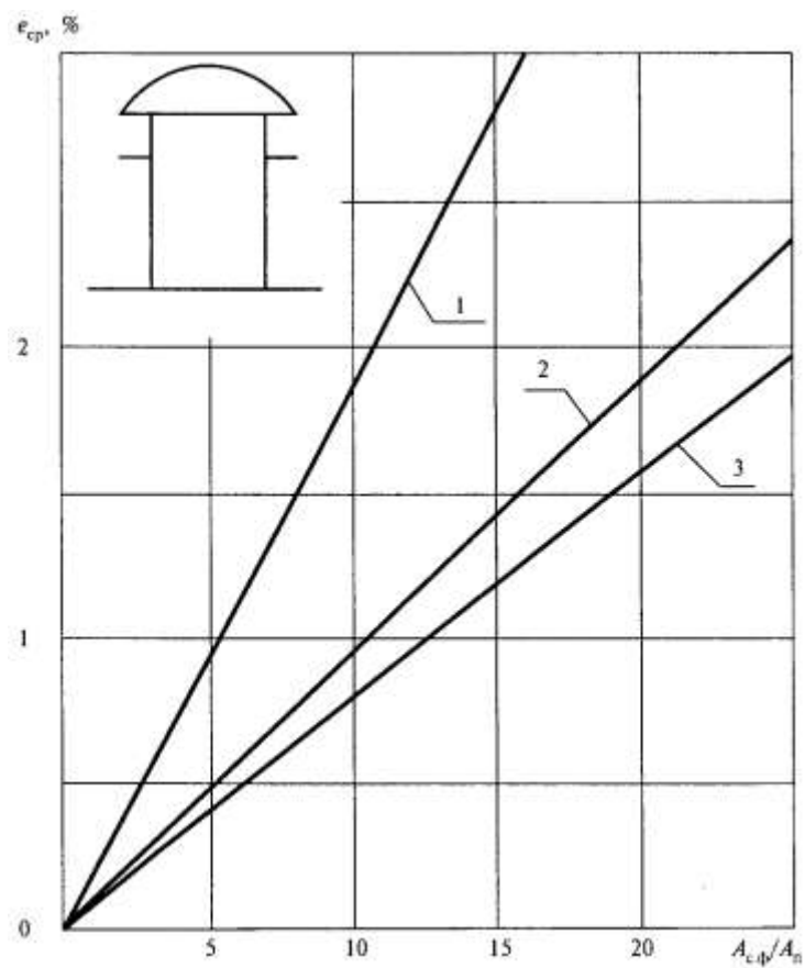
Рисунок 6 — График для определения среднего значения КЕО e_{cp} в общественных помещениях с шахтными фонарями диффузного света с глубиной светопроводной шахты 3,50 м и размерами в плане, м: 1 - 2,9х5,9; 2 - 2,7х 2,7; 2,9х2,9; 1,5х5,9; 3 - 1,5х1,7
