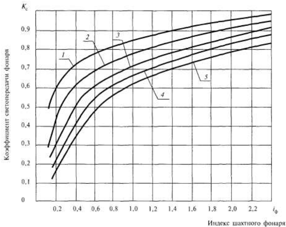
1 - \rho_n = 0,9 ; 2 - \rho_n = 0,8 ; 3 - \rho_n = 0,7 ; 4 - \rho_n = 0,6 ; 5 - \rho_n = 0,5 Рисунок 13 — График для определения коэффициента светопередачи K_c фонарей с направленным отражением стенок шахты при различных значениях коэффициента диффузного отражения стенок шахты
