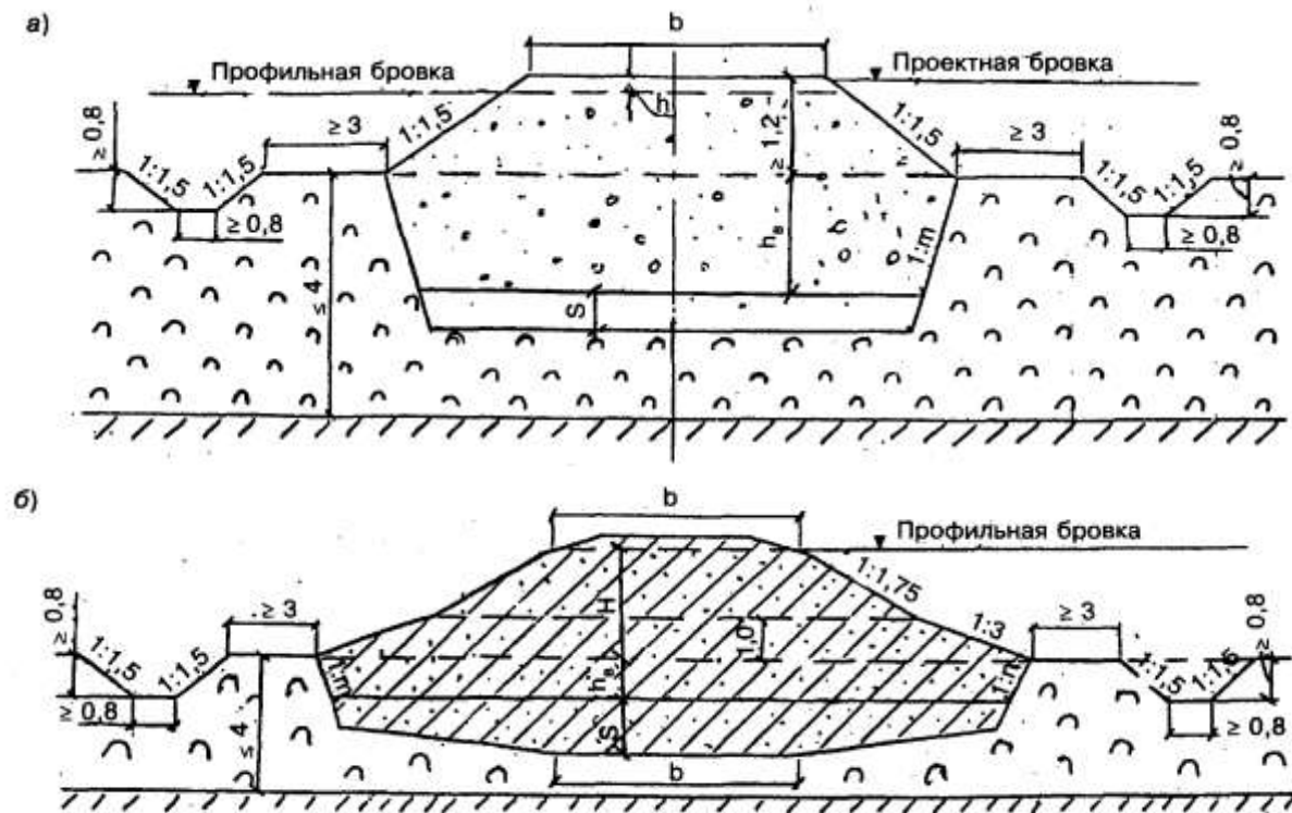
а — из дренирующих грунтов; б — из мелких и пылеватых песков, песчанистых супесей; 1:m — крутизна откосов траншеи выторфовывания (от 1:0 до 1:0,5 ); l , — глубина траншеи выторфовывания; S — осадка насыпи Рисунок 8.2 — Поперечные профили насыпей высотой от 2 до 3 м с частичным выторфовыванием на болотах I типа глубиной от 2 до 4 м при поперечном уклоне минерального дна болота не круче 1:10
