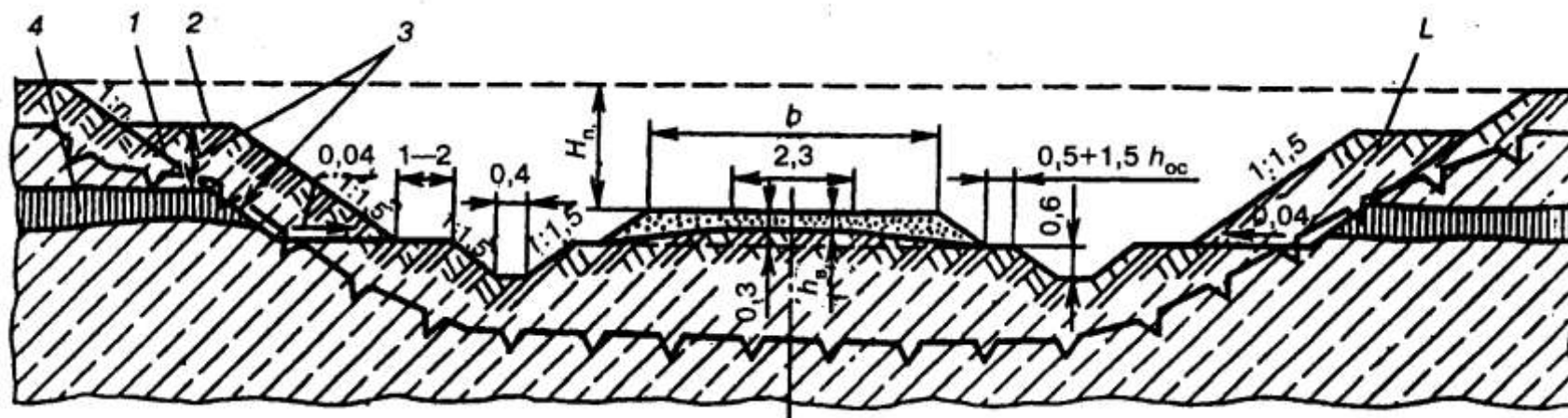
1 — откос не круче 1:1,5; 2 — грунт замены; 3 — расстояние до поверхности слоя льда (не менее двойной глубины оттаивания грунта замены); 4 — лед Рисунок 20.8 — Поперечный профиль выемки, прорезающей слой подземного льда
