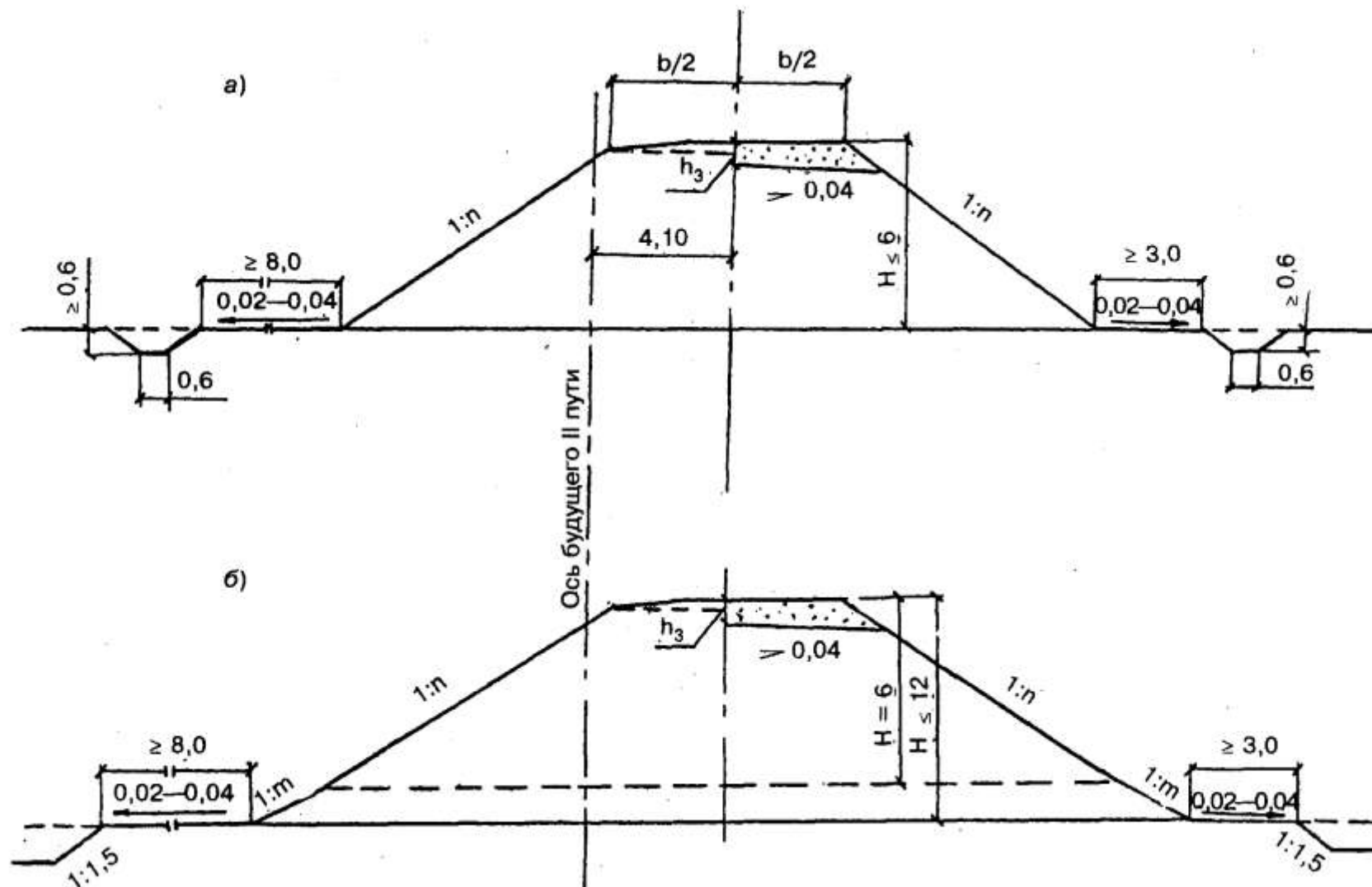
Рисунок 7.1 — Поперечные профили насыпей из недренирующих грунтов при поперечном уклоне местности не круче 1:5
