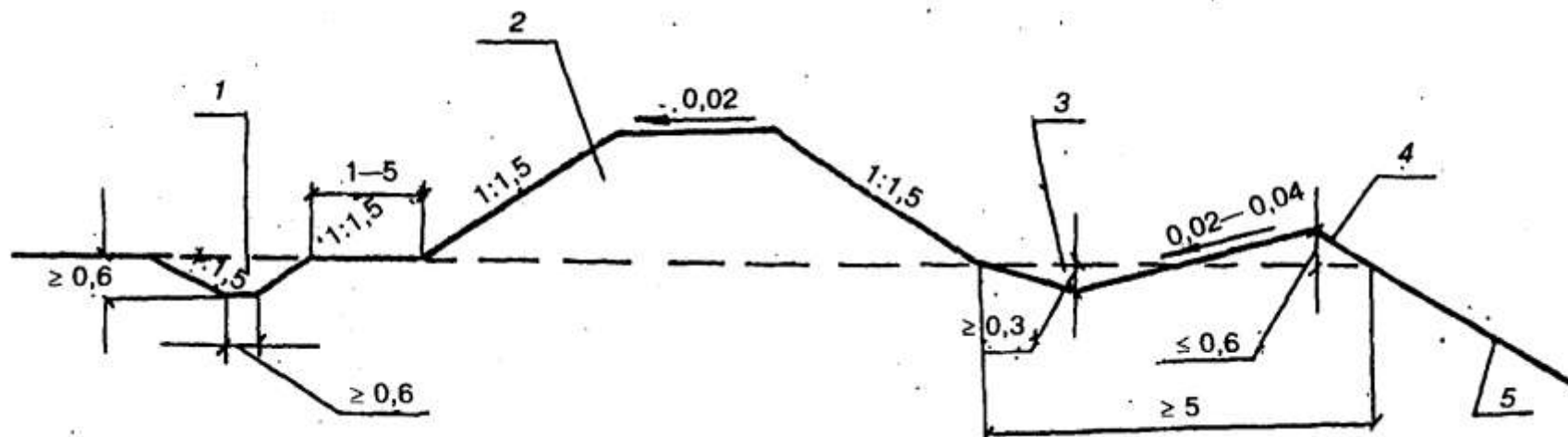
Рисунок 16.1 — Схема размещения банкетов, кавальеров, забанкетных и нагорных канав
