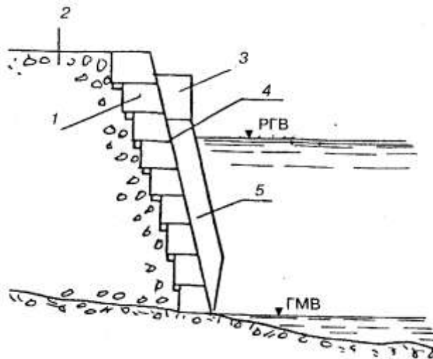
1 — сборная одевающая стена из блоков; 2 — насыпь (или защищаемый берег); 3 — противовес (наращенный участок оседающего массива); 4 — прокладка из толя; 5 — сборно-монолитный оседающий массив
