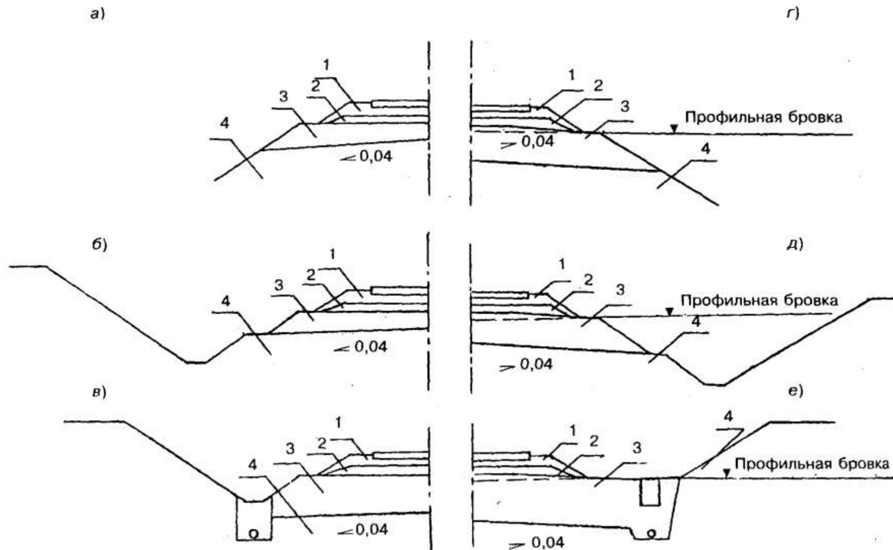
Рисунок 5.2 — Земляное полотно из глинистых грунтов, характеризующихся W_L > 0,23 с защитным слоем
