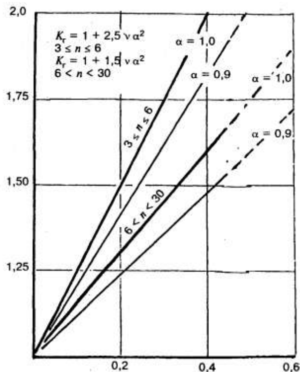
Рисунок Р.4 — График для определения коэффициента безопасности по грунту K_T зависимости от коэффициента вариации v ряда измерений и заданной надежности \alpha
