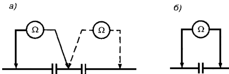
Рисунок 7 - Схема контроля состояния изолирующих фланцев с нейтральной вставкой (а) и без вставки (б)
