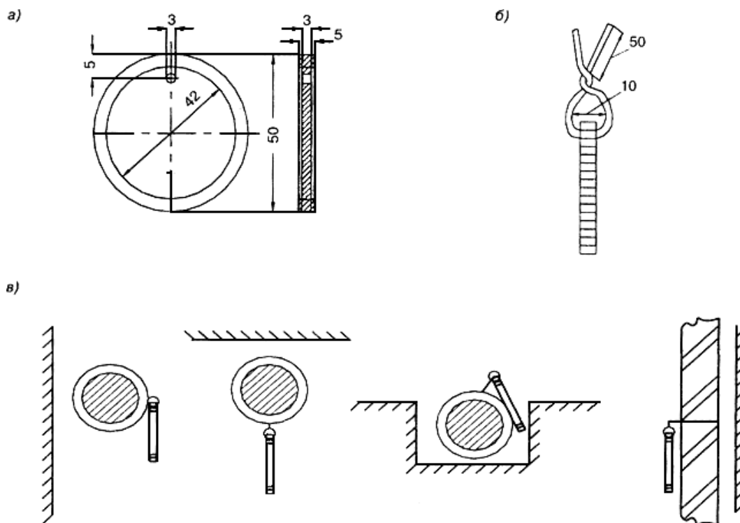
а - общий вид; б - узел подвешивания к проволоке; в - варианты подвешивания к кабелю
