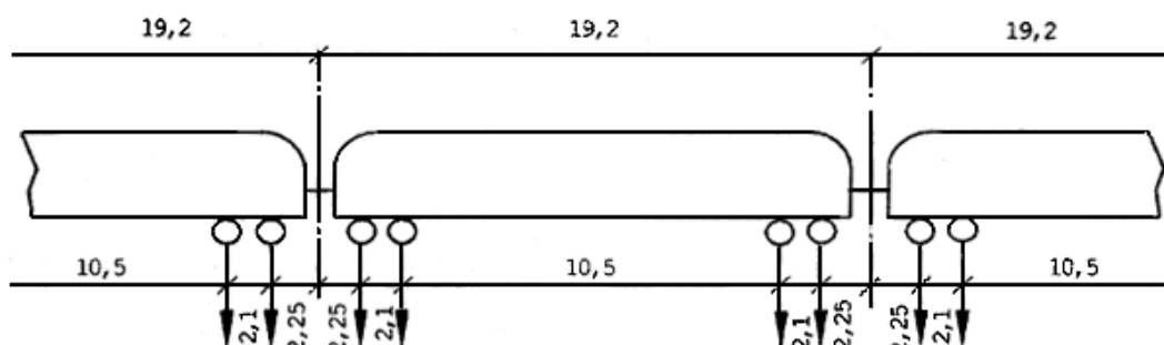
Рисунок 2 - Схема нагрузки на рельсы пути от подвижного состава
