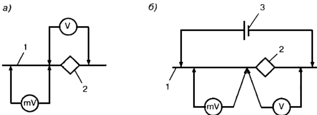
1 - кабель; 2 - изолирующая муфта; 3 - источник тока Рисунок 6 - Схема контроля состояния изолирующих муфт на кабелях приблизительно без источника тока (а) и с источником тока (б)
