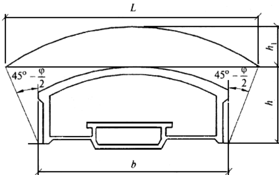
Рисунок 1 - Схема для расчета высоты свода обрушения
