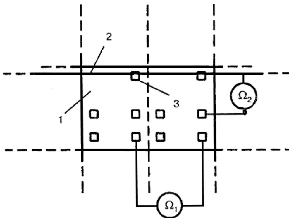
Рисунок 8 - Схема проверки наличия гальванической связи между арматурой железобетонных блоков ( \Omega_1 ), арматурой и шиной заземления ( \Omega_2 )
