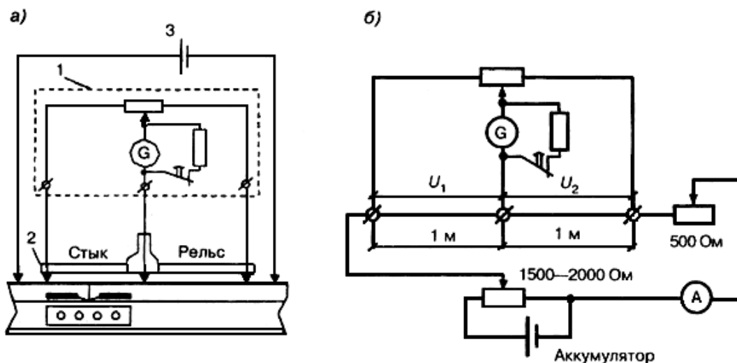
1 - измерительная коробка стыкоизмерителя; 2 - контактная штанга; 3 - источник постоянного тока
