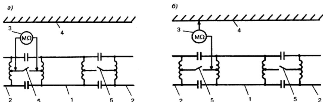
1 - рельсы измеряемого участка; 2 - рельсы смежных участков; 3 - измерительный прибор; 4 - обделка тоннеля; 5 - отсоединенная средняя шина
