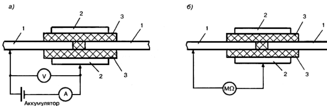
1 - рельс; 2 - путевая накладка; 3 - изолирующие конструктивные элементы Рисунок 5 - Схема измерения сопротивления изоляции стыка ходового рельса
