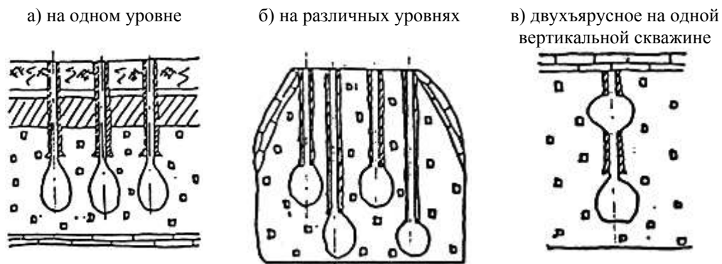
Рисунок 1 - Расположение выработок-емкостей
