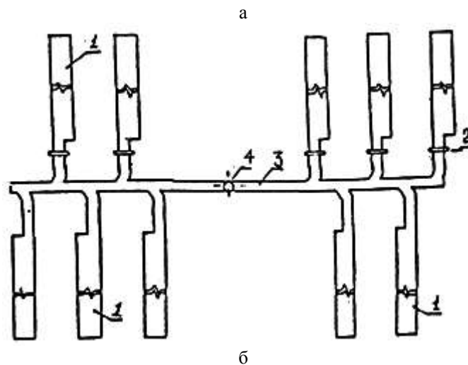
Рисунок 3 - Вскрывающие выработки
