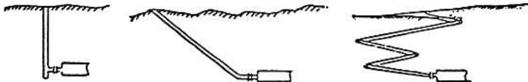
Рисунок 3 - Вскрывающие выработки
