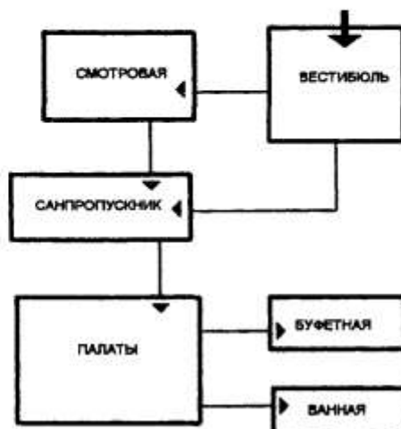
СХЕМА ВЗАИМОСВЯЗИ ПОМЕЩЕНИЙ
