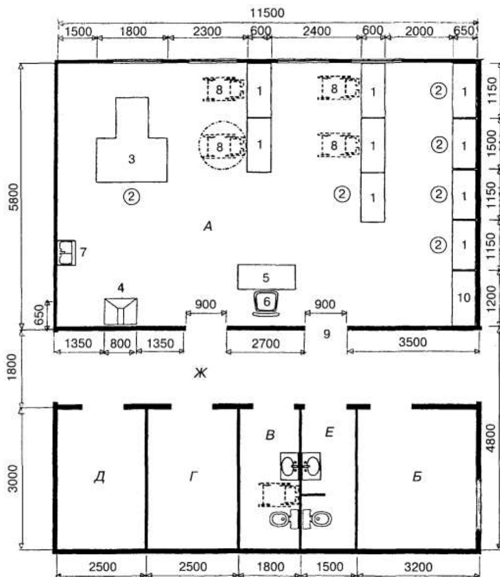
Планировочная схема картонной мастерской
