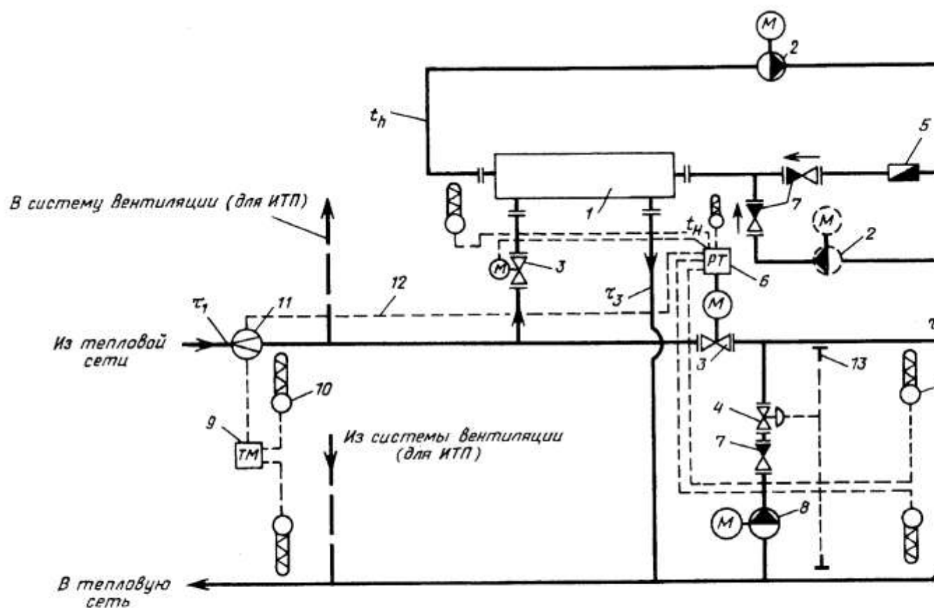
Рис. 1. Одноступенчатая система присоединения водоподогревателей горячего водоснабжения с автоматическим регулированием расхода теплоты на отопление и зависимым присоединением систем отопления в ЦТП и ИТП 1 — водоподогреватель горячего водоснабжения; 2 — повысительно-циркуляционный насос горячего водоснабжения (пунктиром обозначен регулируемый клапан с электроприводом); 3 — регулятор перепада давлений (прямого действия); 4 — водомер для холодной воды; 5 — регулятор горячего водоснабжения и ограничения максимального расхода сетевой воды на ввод; 6 — обратный клапан; 7 — корректирующий клапан; 8 — датчик температуры; 9 — датчик расхода воды; 10 — датчик температуры; 11 — датчик расхода воды; 12 — сигнал ограничения максимального расхода воды из тепловой сети в трубопроводе
