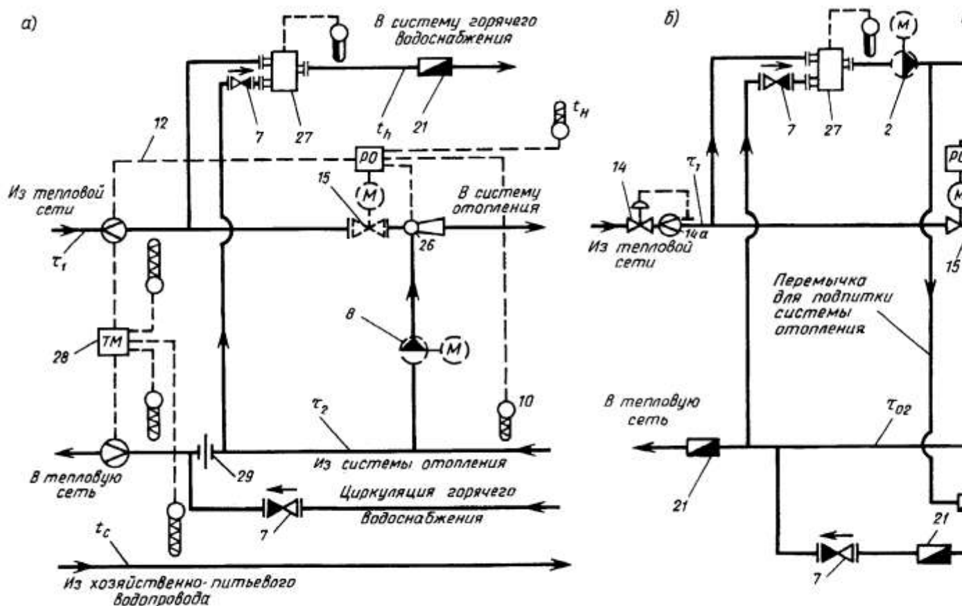
Рис. 9. Схемы присоединения систем горячего водоснабжения и отопления в ИТП при зависимом (а) присоединении систем (пунктиром — с циркуляционным насосом) с учетом теплоты по тепломеру и независимом (б) — с учетом теплоты по водомеру
