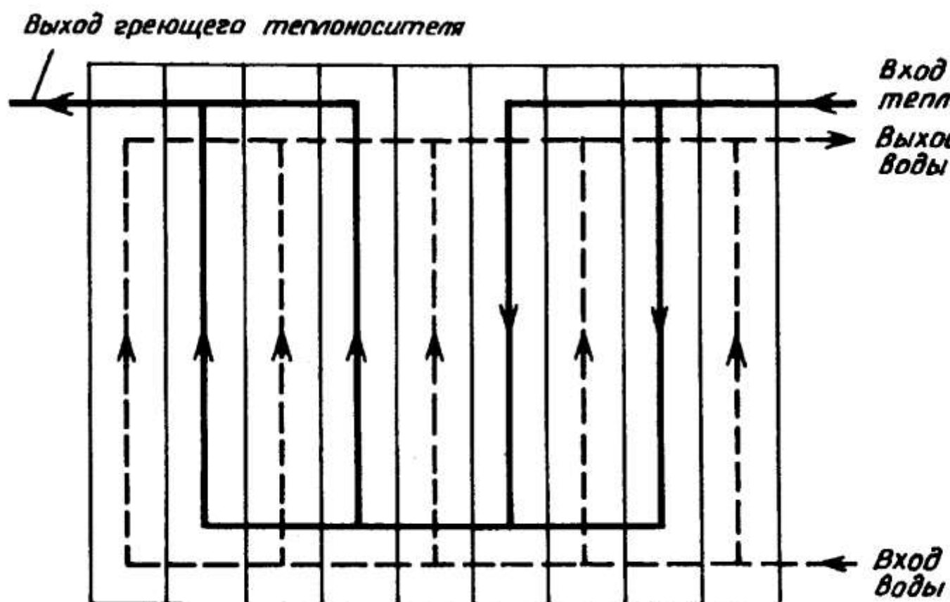
Рис. 2. Несимметричная компоновка пластинчатого водоподогревателя, обозначение
