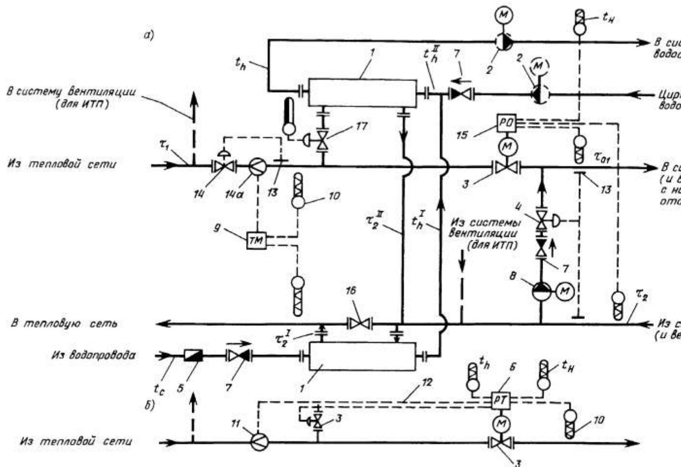
Рис. 2. Двухступенчатая схема присоединения водоподогревателей горячего водоснабжения для жилых и общественных зданий и с зависимым присоединением систем отопления в ЦТП и ИТП
