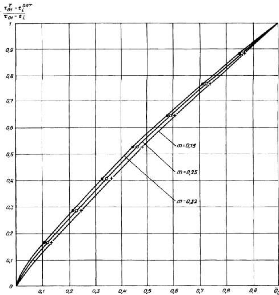
Рис. 2. Графики изменения температурного критерия системы отопления по температуре воды в подающем трубопроводе \frac{\tau_{01} - t_i^{opt}}{\tau_{01} - t_i} для различных значений показателя степени m и при постоянной циркуляции теплоносителя в системе
