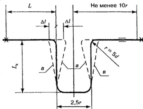
Рисунок 10 - Диаграмма для определения удлинения труб
