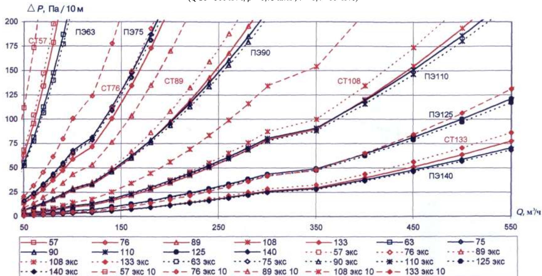
Удельные потери давления для стальных и полиэтиленовых труб (новых и бывших в эксплуатации) низкого давления ( Q 50 - 500 м 3 /ч, \rho = 0,73 кг/м 3 , \nu = 1,4 \cdot 10^{-6} м 2 /с)
