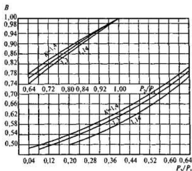
Рисунок 6— Зависимость коэффициента B от P_2 / P_1 .
