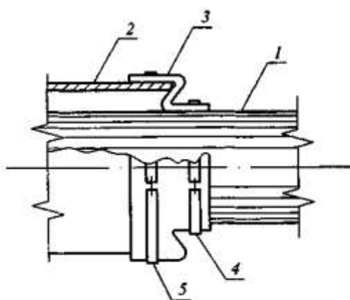
Рисунок 3 — Прокладка газопровода в футляре
