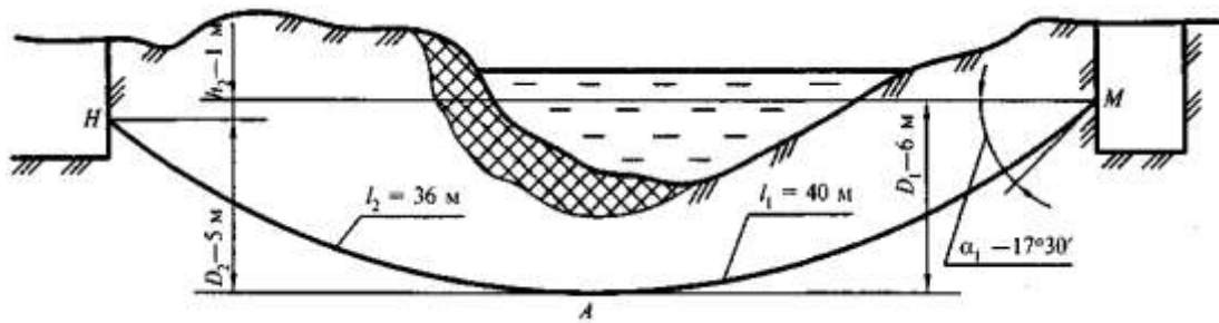
Рисунок Л.4 — Расчетные параметры пилотной скважины
