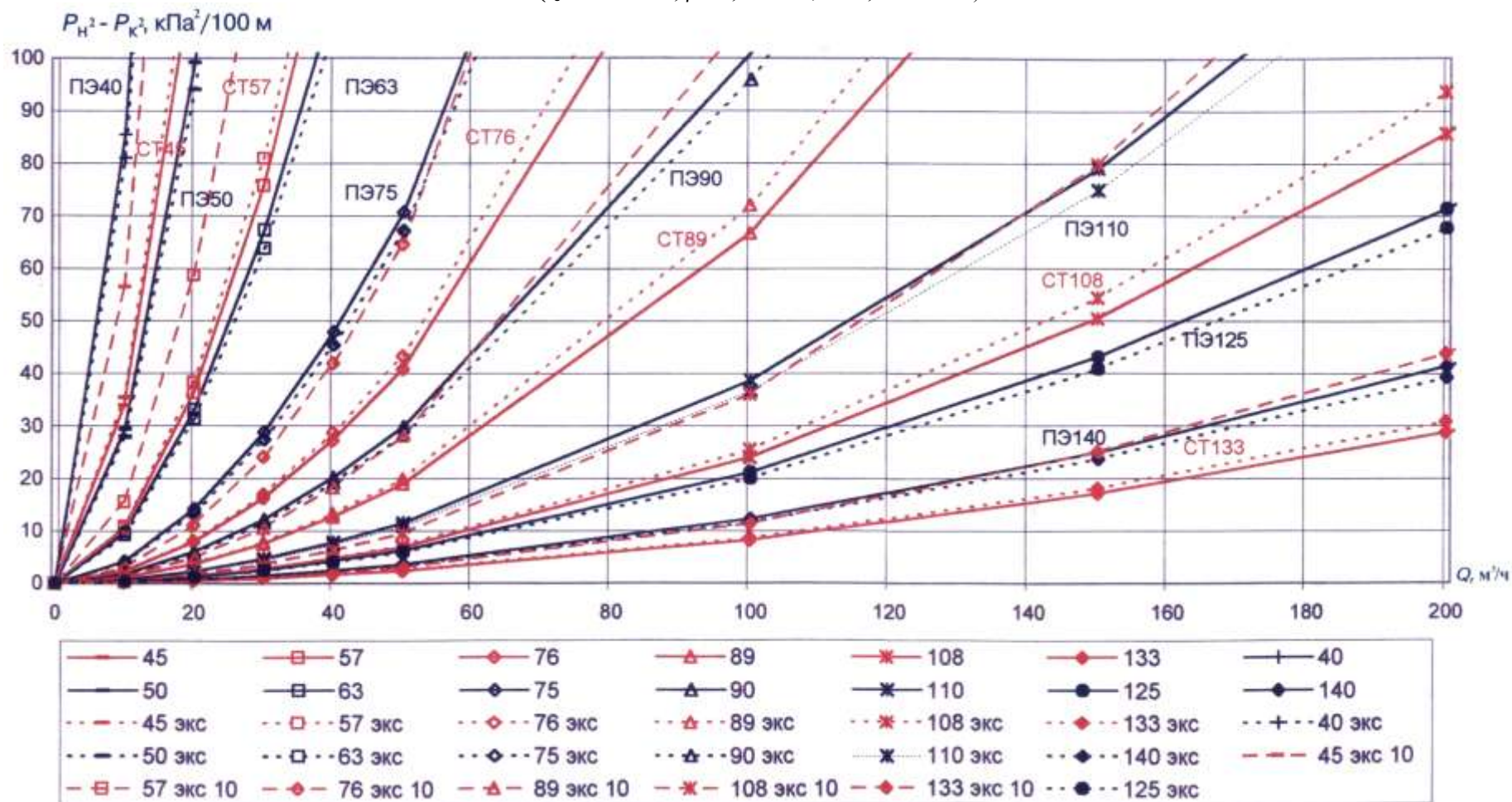
Удельные потери давления для стальных и полиэтиленовых труб (новых и бывших в эксплуатации) высокого давления ( Q 0 - 200 м 3 /ч, \rho = 0,73 кг/м 3 , \nu = 1,4 \cdot 10^{-6} м 2 /с)
