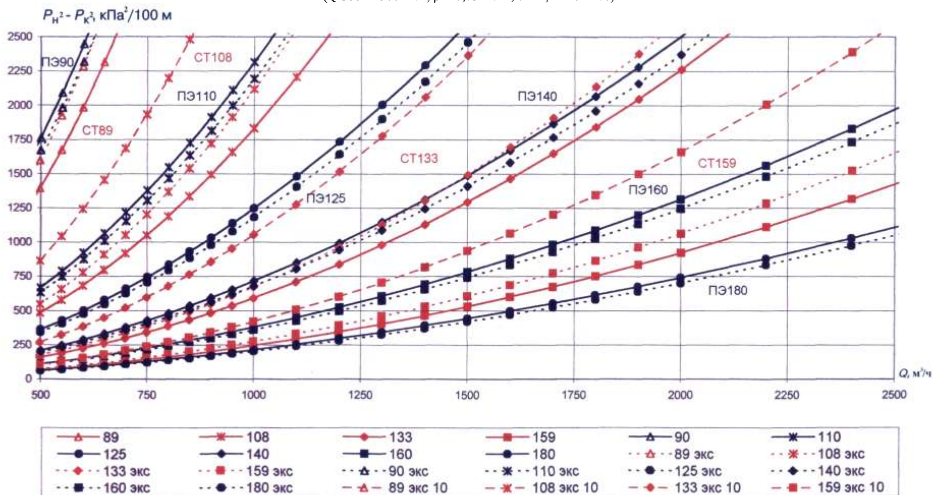
Удельные потери давления для стальных и полиэтиленовых труб (новых и бывших в эксплуатации) высокого давления ( Q 500 - 2500 м 3 /ч, \rho = 0,73 кг/м 3 , \nu = 1,4 \cdot 10^{-6} м 2 /с)
