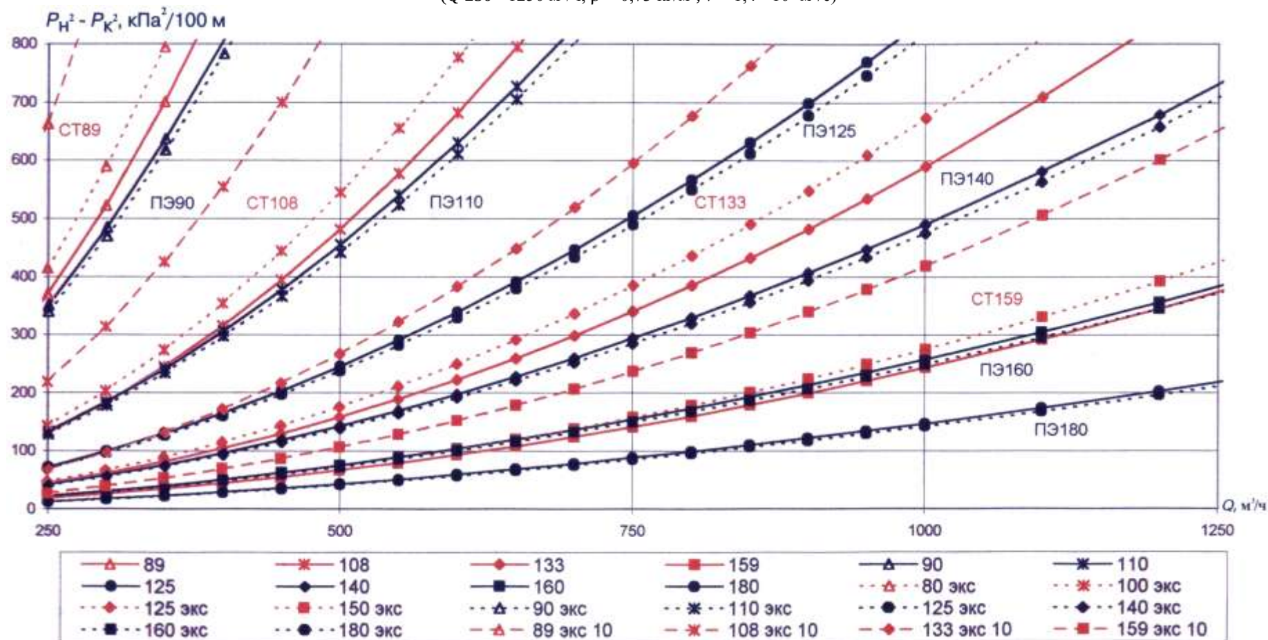
Удельные потери давления для стальных и полиэтиленовых труб (новых и бывших в эксплуатации) низкого давления ( Q 250 - 1250 м 3 /ч, \rho = 0,73 кг/м 3 , \nu = 1,4 \cdot 10^{-6} м 2 /с)
