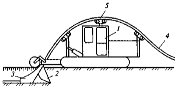
1 — гусеничный тягач; 2 — режущий нож; 3 — щелезасыпщик; 4 — трубная плеть; 5 — роликоопоры
