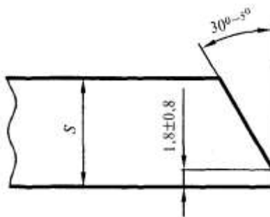
Рисунок 9 — Схема обработки кромки
