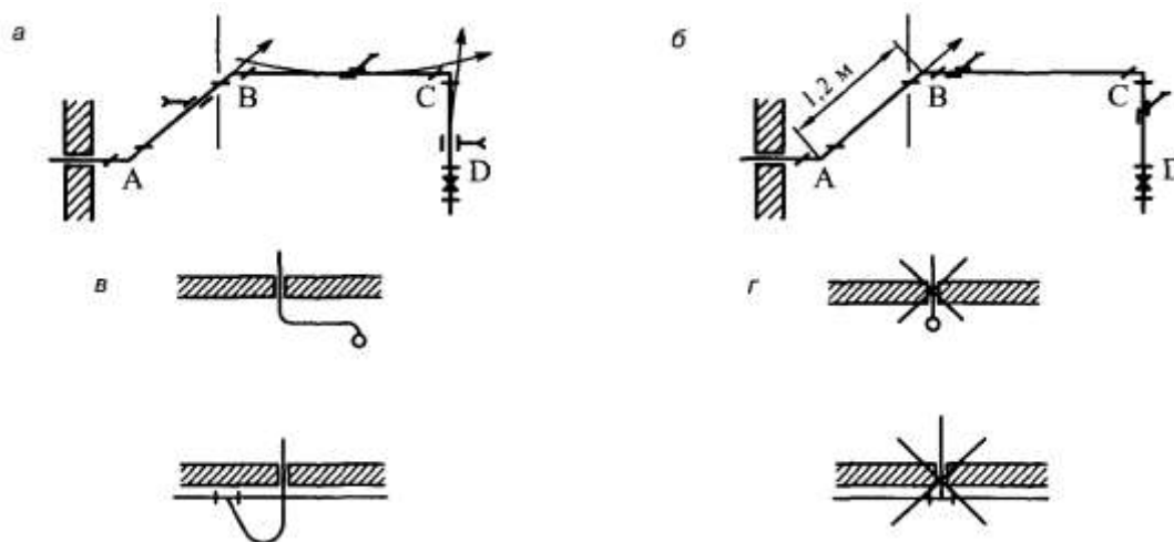
Рисунок 7 — Прокладка газопроводов с соблюдением правил естественной компенсации а — правильная прокладка газопровода; б — неправильная прокладка газопровода; в — правильная прокладка ответвления газопровода; г — неправильная прокладка ответвления газопровода
