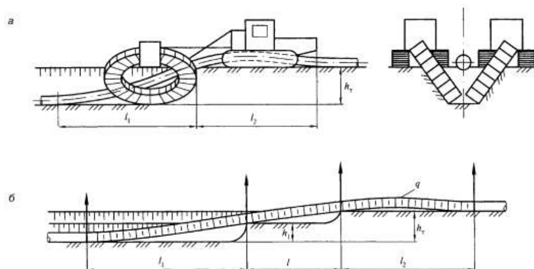
Рисунок 23 — Укладка газопровода методом «подкопа»
