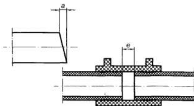
a — максимальный допуск косого среза трубы; e — максимальный зазор между двумя концами труб в муфте
