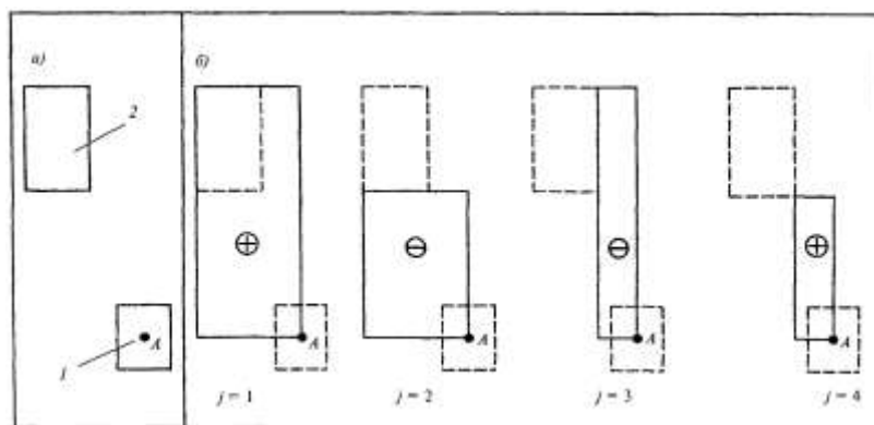
a - схема расположения рассчитываемого 1 и влияющего фундамента 2; b - схема расположения фиктивных фундамента с указанием знака напряжений \sigma_{zp,cj} в формуле (5.19) под углом j -го фундамента
