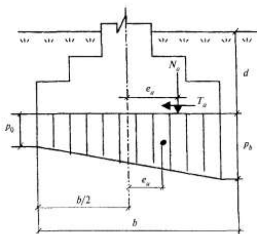
Рисунок 6.10 - Эпюра предельного давления под подошвой фундамента при сейсмическом воздействии
