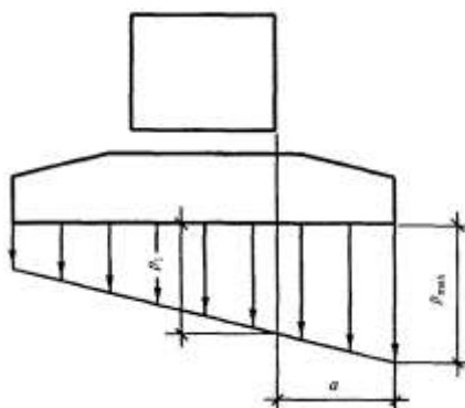
Рисунок 12.2 - К расчету ленточного фундамента
