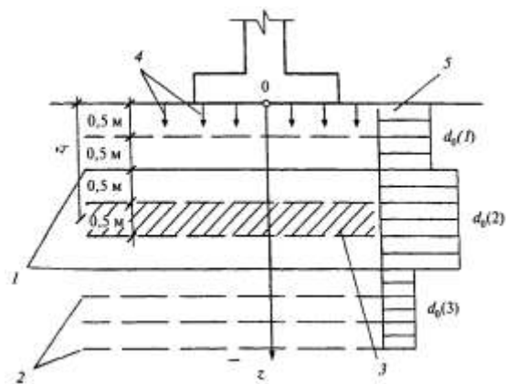
1 - границы слоев с различным содержанием гипса; 2 - границы расчетных слоев; 3 - расчетный слой; 4 - направление фильтрации; 5 - начальная эпюра относительного содержания гипса d_0(z)
