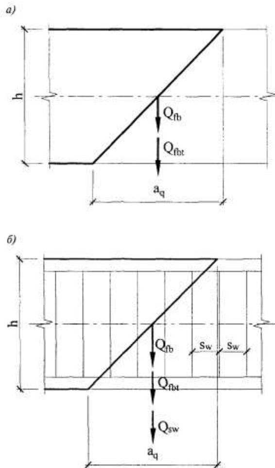
a — при фибровом армировании; b — при комбинированном армировании
