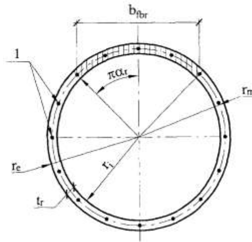
1 — стержневая арматура
