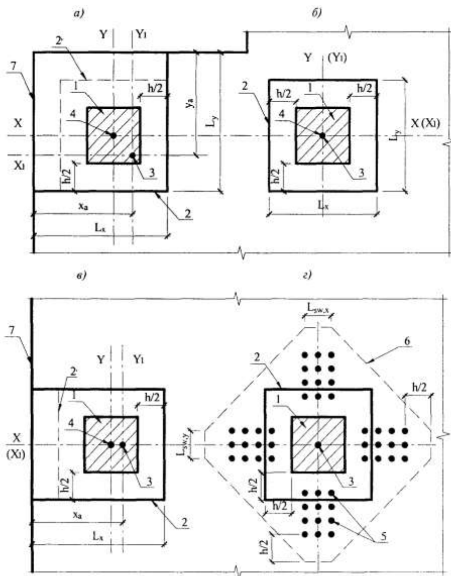
a, в — площадка приложения нагрузки у края плоского элемента; б — то же, внутри плоского элемента; г — при крестообразном расположении поперечной арматуры; 1 — площадь приложения нагрузки; 2 — расчетный контур поперечного сечения; 2' — второй вариант расположения расчетного контура; 3 — центр тяжести расчетного контура (место пересечения осей X_1 и Y_1 ); 4 — центр тяжести площадки приложения нагрузки (место пересечения осей X и Y ); 5 — поперечная арматура; 6 — контур расчетного поперечного сечения без учета в расчете поперечной арматуры; 7 — группа (край) плоского элемента
