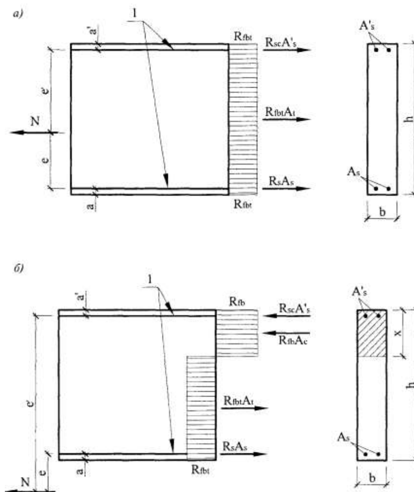
a — между равнодействующими усилий в арматуре S и S' ; b — за пределами расстояния между равнодействующими усилий в арматуре S и S' ; 1 — стержневая арматура
