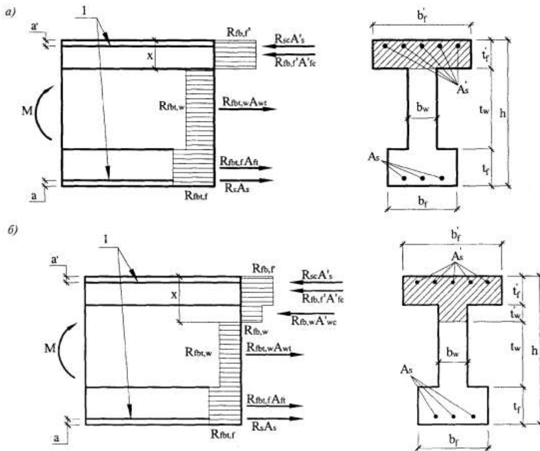
a — при x \leq t'_f ; б — при x > t'_f ; 1 — стержневая арматура
