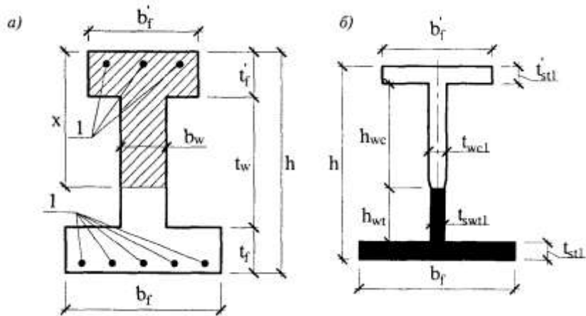
a — сечение сталефибробетонного элемента; б — сечение, приведенное к стальному; 1 — стержневая арматура
