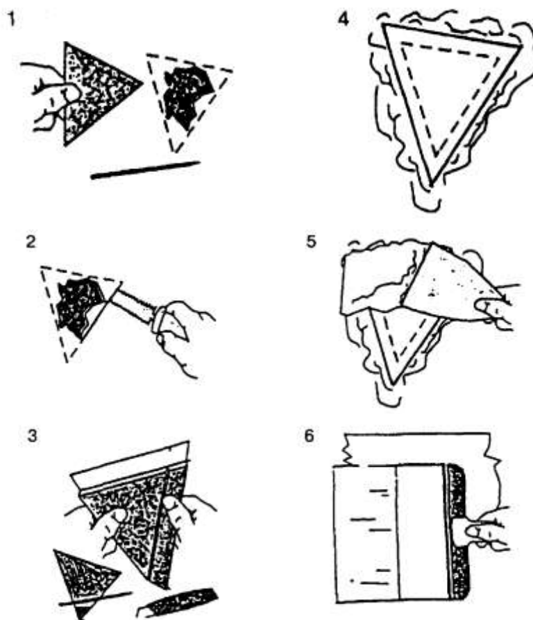
Рисунок 45 — Последовательность операций по заделке малых пробоин в ГКЛ
