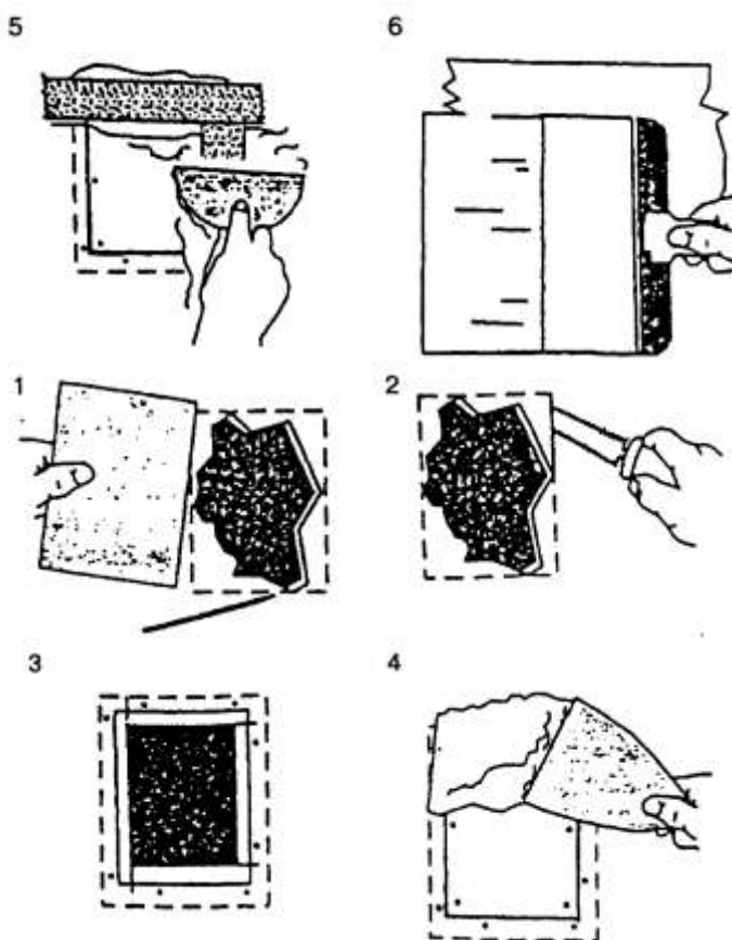
Рисунок 46 — Последовательность операций по заделке больших пробоин в ГКЛ
