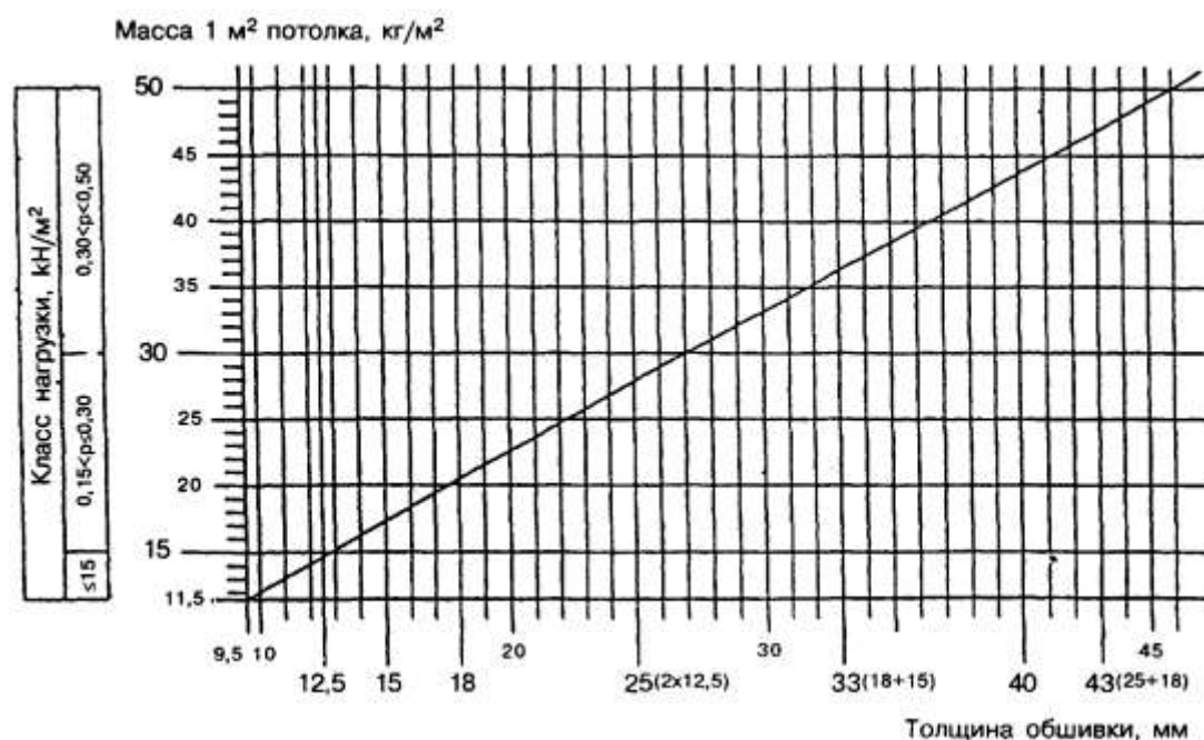
Рисунок 31 — График для определения класса нагрузки подвесного потолка
