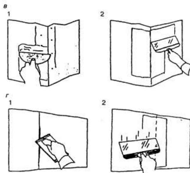
Рисунок 49 — Последовательность операций по заделке трещин на внутренних углах (а), на ленте, наложенной на стык (б), на угловой защитной накладке (в) и по заделке выступов на стыках ГКЛ (г)
