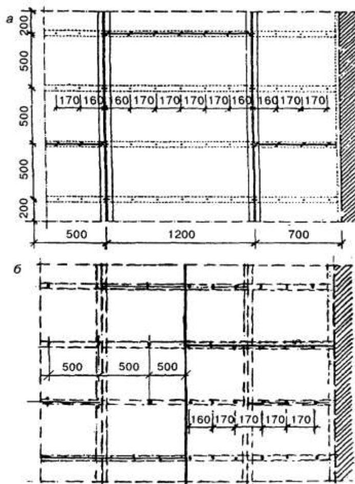
Рисунок 33 — Схемы размещения шурупов крепления однослойной (а) и двухслойной (б) обшивки в подвесных потолках
