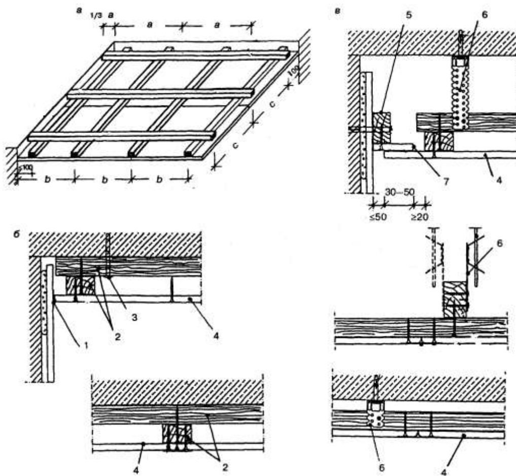
1 — разделительная лента; 2 — бруски каркаса; 3 — анкерный элемент; 4 — обшивка из ГКЛ; 5 — брусок; 6 — подвес; 7 — полоса из ГКЛ
