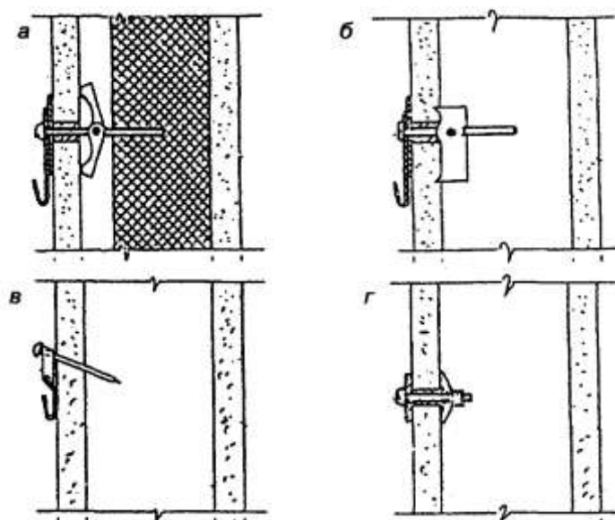
Рисунок 16 — Конструктивные решения навески предметов на обшивку из гипсокартонных листов перегородок с применением анкеров (а, б), крючков (в) и дюбелей (г)
