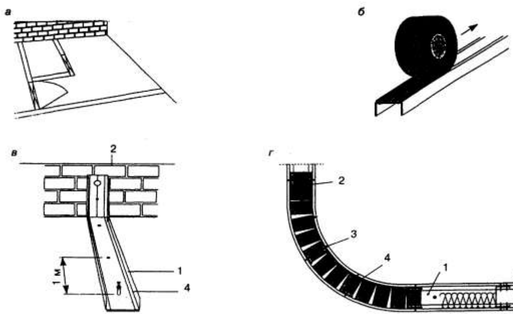
Рисунок 40 — Конструкция шаблона (а), схема гнутья ГКЛ (б) и общий вид игольчатого валика (в)
