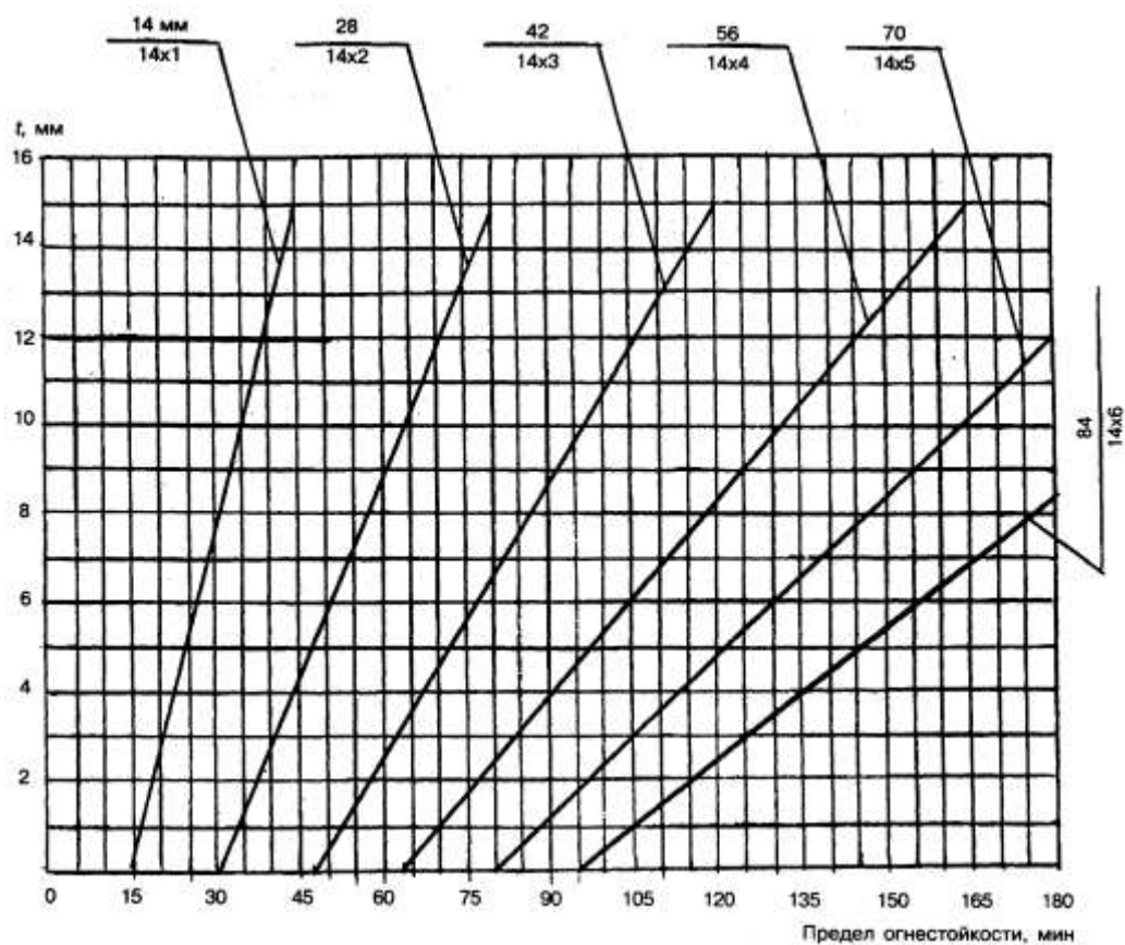
Рисунок 38 — Зависимость предела огнестойкости стальных конструкций от количества слоев ГКЛ и приведенной толщины стали t
