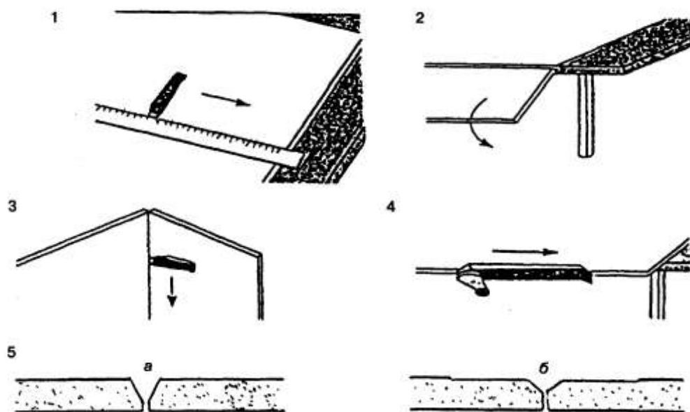
1 — резка; 2 — надлом; 3 — разрезка картона на обратной стороне ГКЛ; 4 — обработка обрезанной кромки рубанком; 5 — подготовка обрезанной кромки под шпаклевку шва с армирующей лентой
