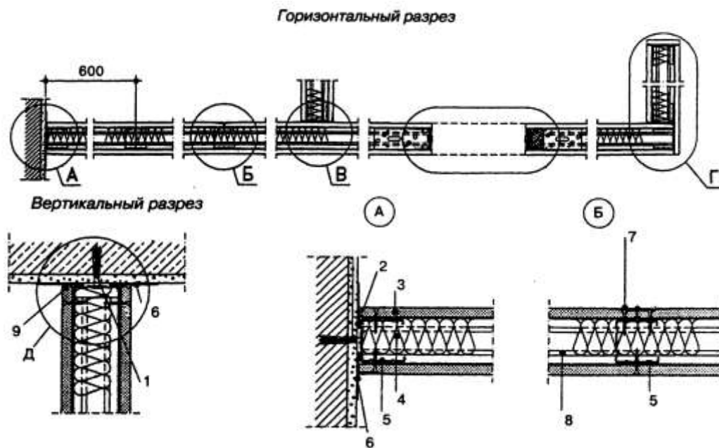
Рисунок 9 — Места установки уплотнительной ленты в конструкции перегородок из гипсокартонных листов
