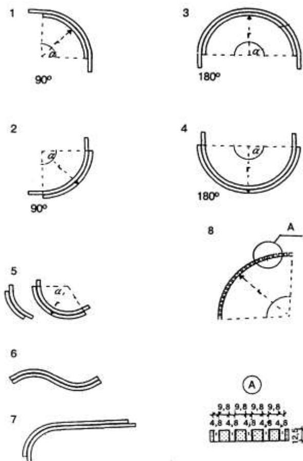
Рисунок 3 — Варианты гипсокартонных элементов
