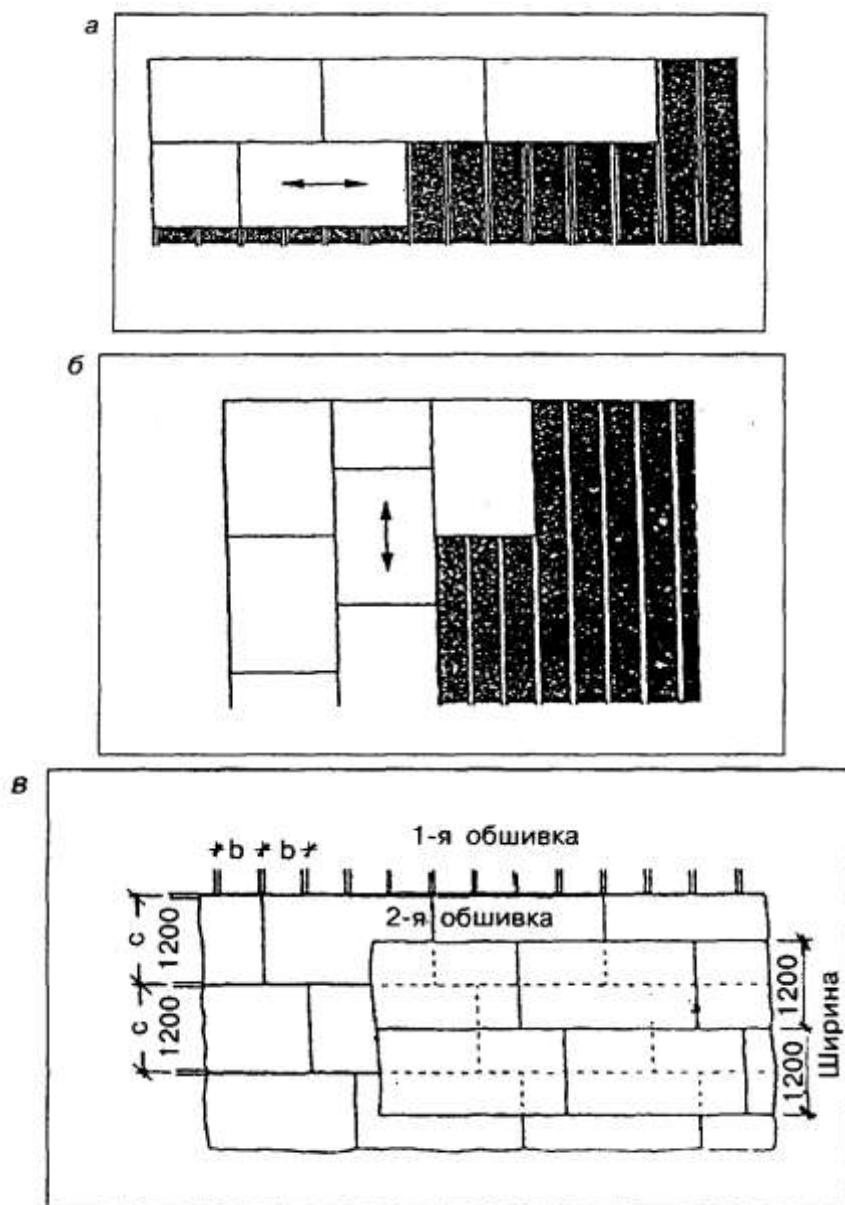
Рисунок 32 — Схемы размещения гипсокартонных листов в подвесных потолках поперек несущих профилей (а), вдоль несущих профилей (б) и смещения листов при двухслойной обшивке (в)
