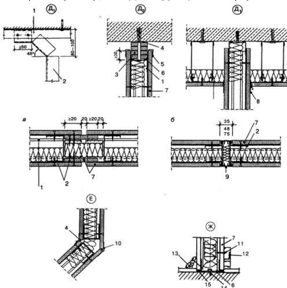
Рисунок 10 — Конструктивные решения узлов перегородки из гипсокартонных листов с примыканием к стене (А), стыка гипсокартонных листов (Б), Т-образного сопряжения (В), образования угла и торца стены (Г). Узлы (Д, Е, Ж) показаны на рисунке 11
