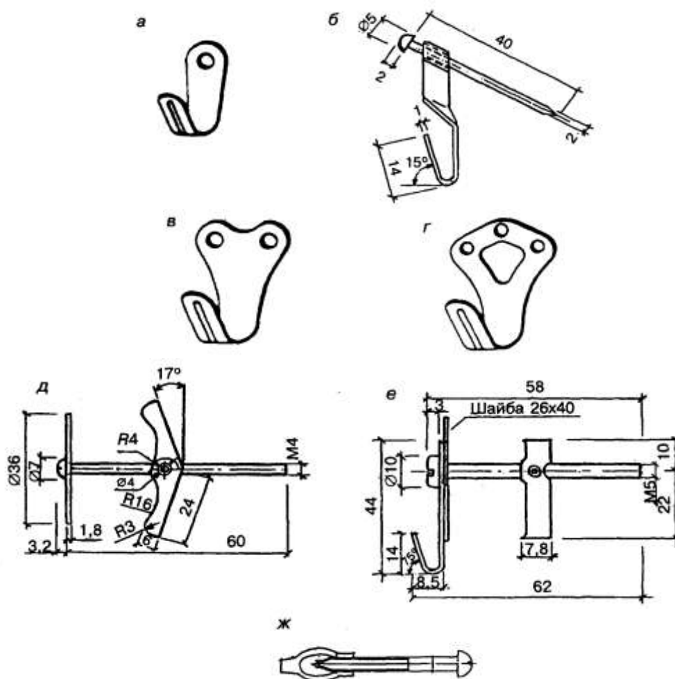
Рисунок 7 - Крючки (а-г), анкеры (д, е) и дюбели (ж) для навески на перегородки из гипсокартонных листов предметов (картин и т.п.) и оборудования массой: а — до 5 кг; б — до 5 кг (по ТУ 400-28-371); в—до 10 кг; г — до 15 кг; д— 30-40 кг (по ТУ 400-28-369); е— 20-30 кг (по ТУ 400-28-370); ж — 20 кг (по ТУ 36-941)
