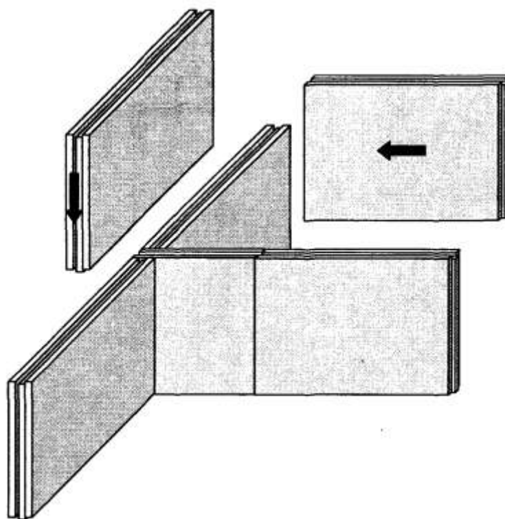
Рисунок 14 — Схема раскладки плит в узле пересечения перегородок
