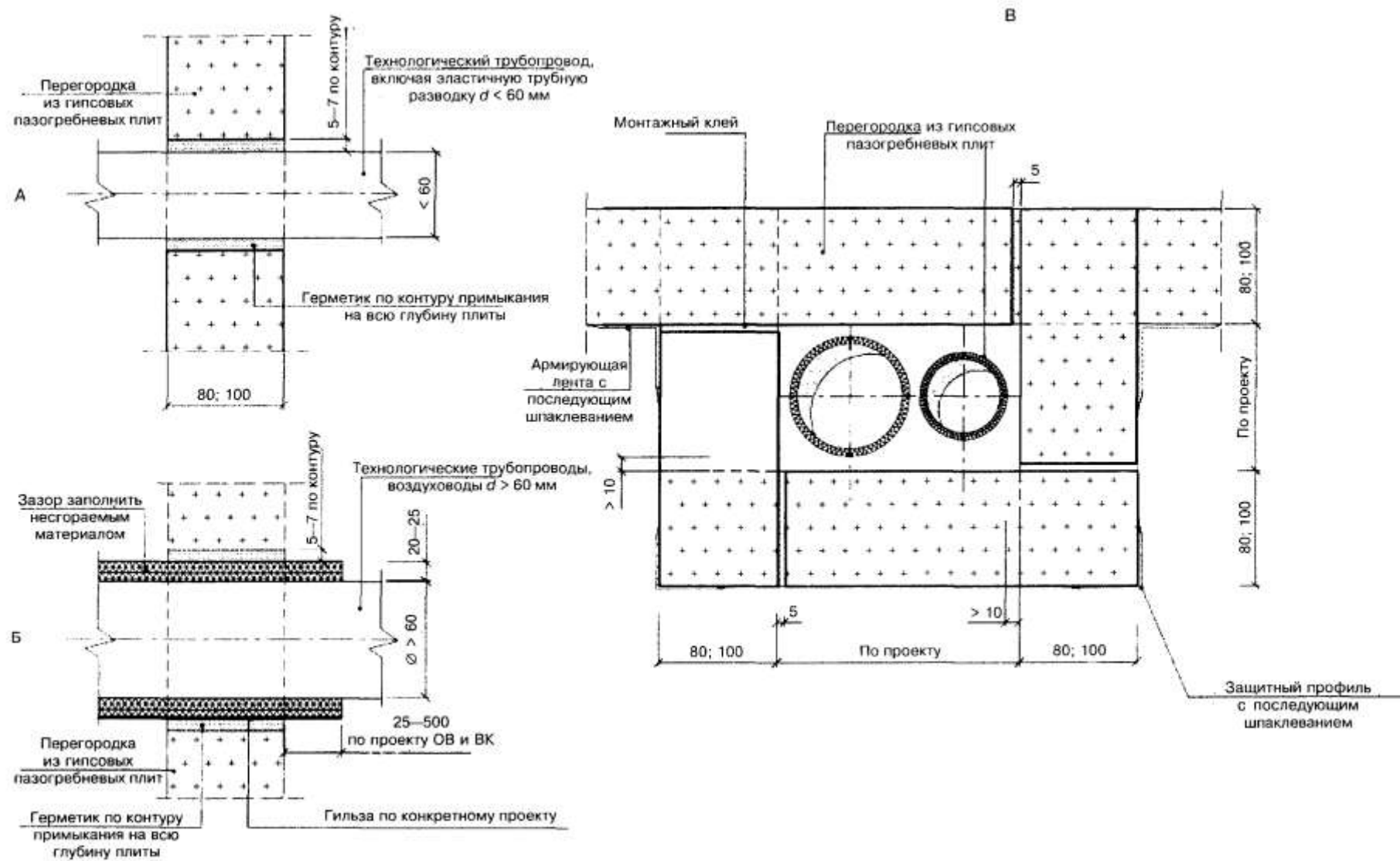
Рисунок 8 — Конструкции узлов пропуска трубопроводов диаметром до 60 мм (А) и более (Б) через перегородку и через шахту (В)
