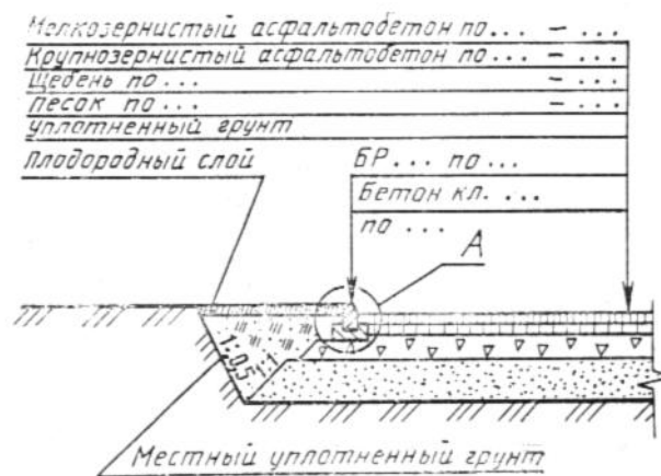
Тротуар (тип 2)
