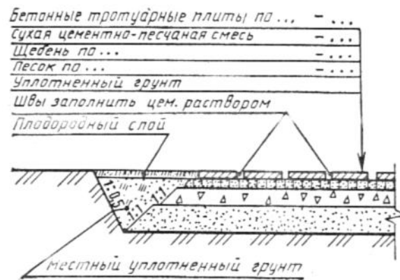
Тротуар (тип 2)
